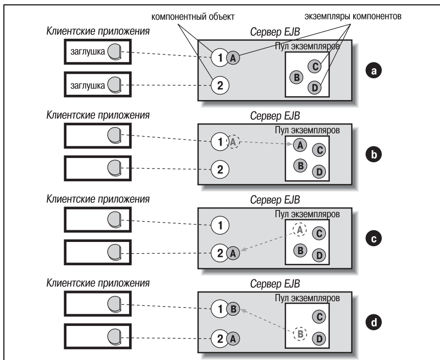
Рис. 3.3. Сеансовые компоненты без состояния и стратегия подкачки
