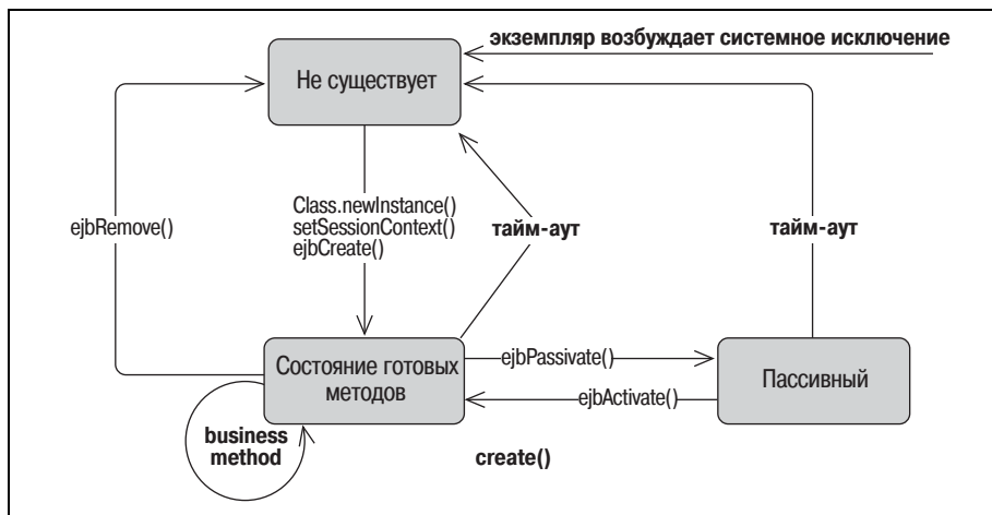
Рис. 12.2. Жизненный цикл сеансового компонента с состоянием
