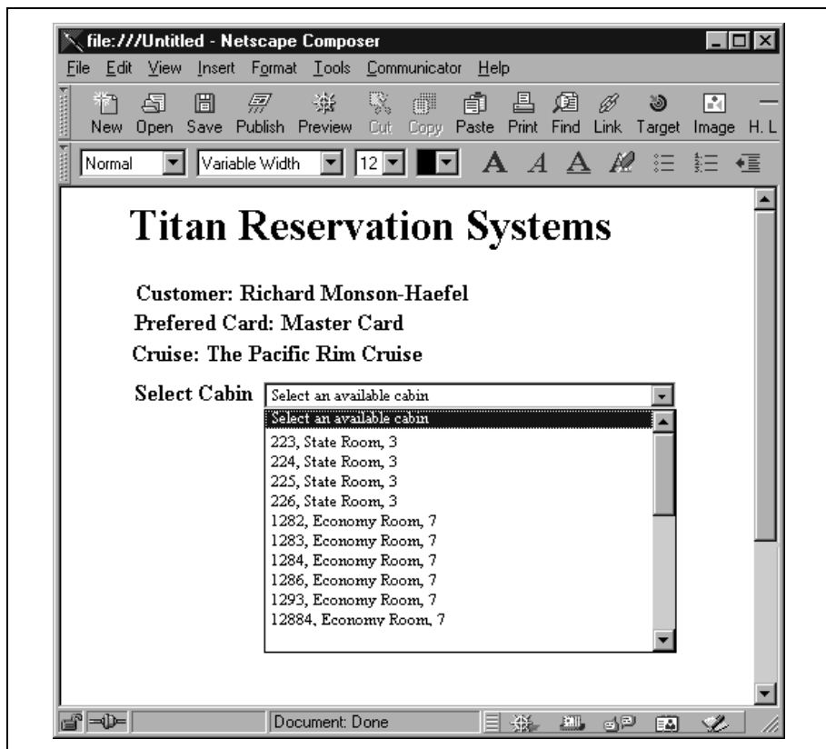
Рис. 17.5. Интерфейс HTML для системы резервирования «Титан»
