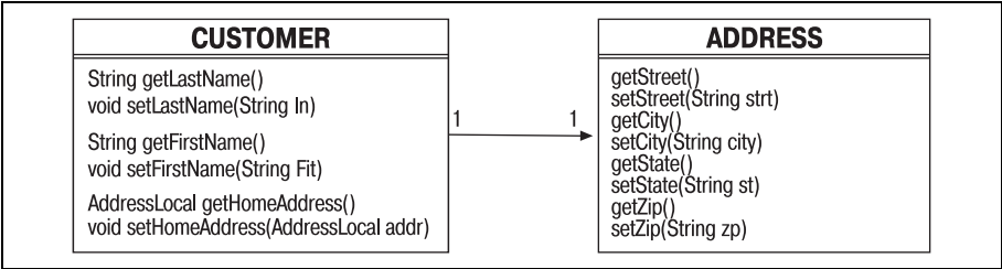
Рис. 7.1. Однонаправленное отношение «один-к-одному»
