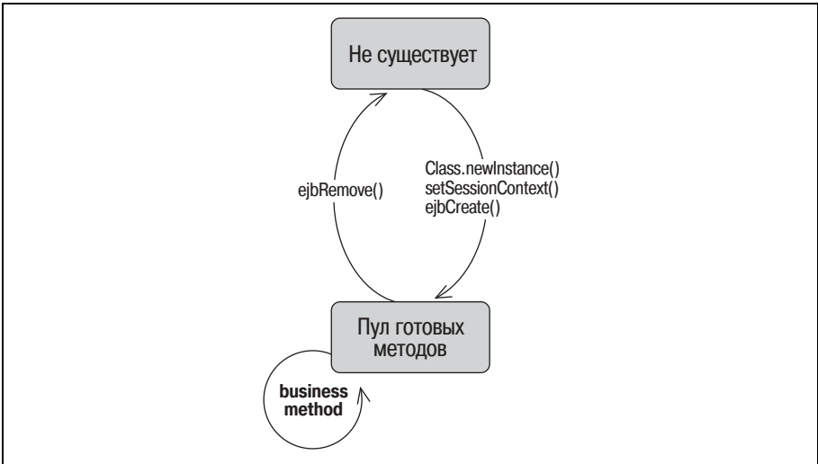
Рис. В.6. Диаграмма состояний жизненного цикла сеансового компонента без состояния
