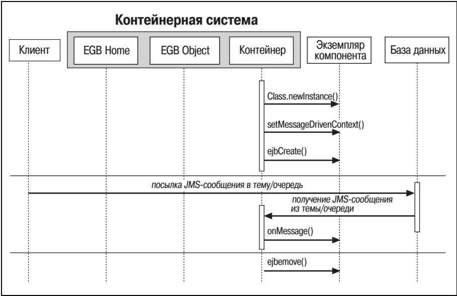
Рис. В.14. Диаграмма последовательностей компонента, управляемого сообщениями
