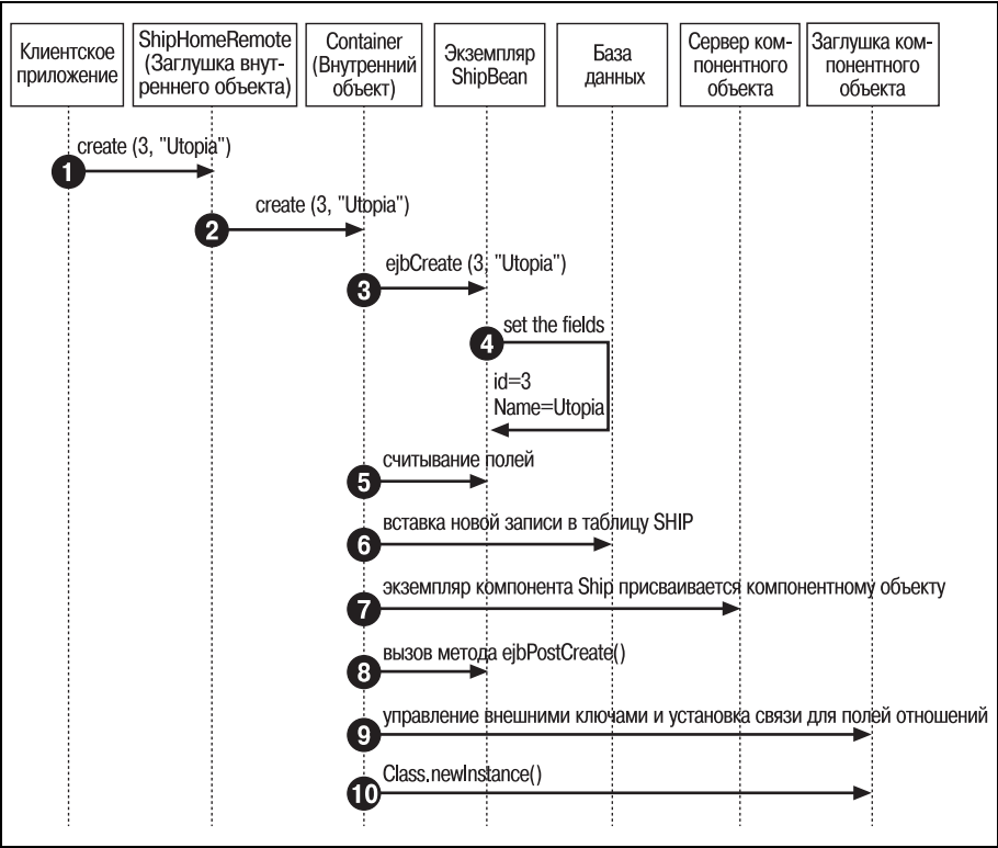
Рис. 11.1. Последовательность создания экземпляра компонента
