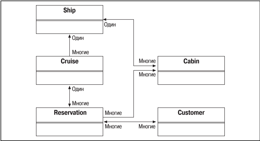
Рис. 7.10. Диаграмма классов Cruise, Ship, Reservation, Cabin и Customer
