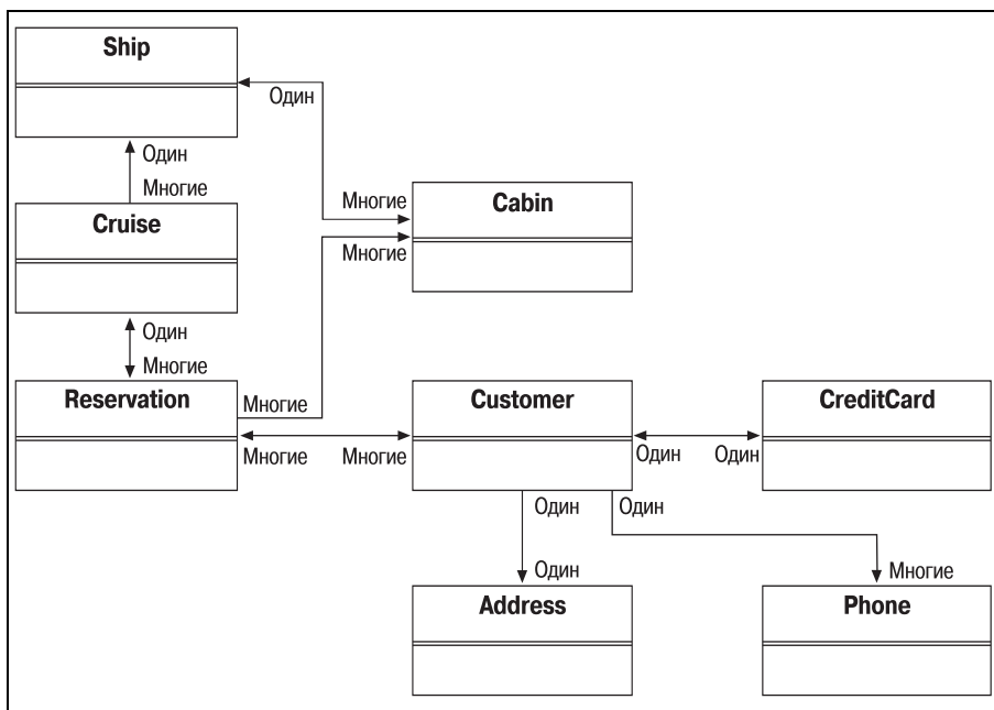
Рис. 8.1. Диаграмма классов «Titan Cruise»
