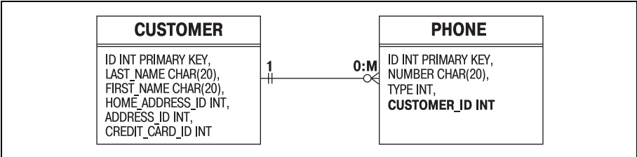
Рис. 7.6. Одностороннее отношение «один-ко-многим» в СУРБД с использованием обратных указателей
