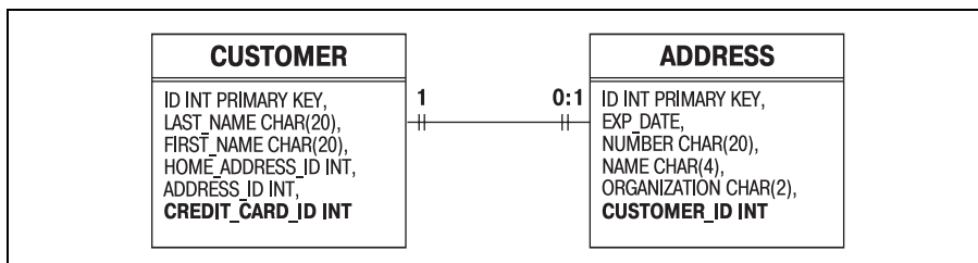
Рис. 7.4. Двухнаправленные отношения «один-к-одному» в СУРБД
