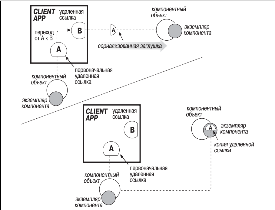
Рис. 5.2. Параметры в виде удаленной ссылки в Java RMI
