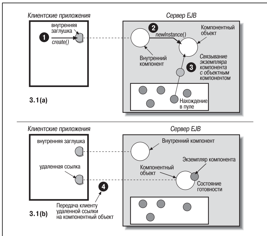
Рис. 3.1. Компонент перемещается из пула экземпляров в состояние готовности
