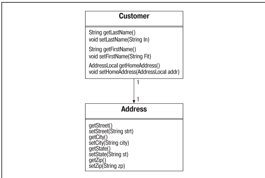
Рис. 6.1. Диаграмма классов компонентов Customer и Address
