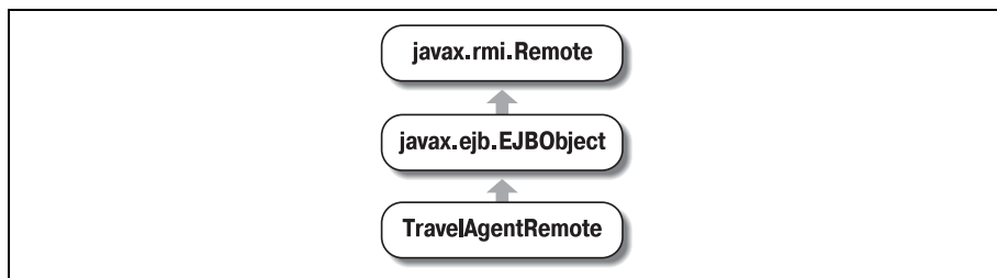
Рис. 5.4. Иерархия наследования интерфейсов компонента
