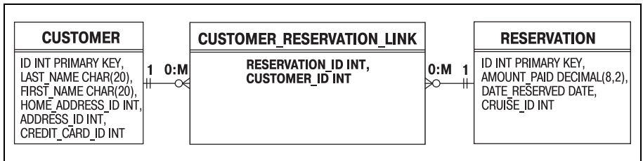
Рис. 7.16. Двухнаправленное отношение «многие-ко-многим» в СУРБД
