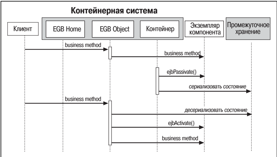
Рис. В.11. Процесс активации сеансовых компонентов с состоянием
