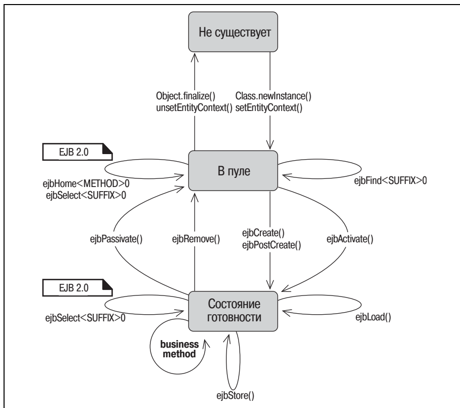
Рис. 11.2. Жизненный цикл объектного компонента
