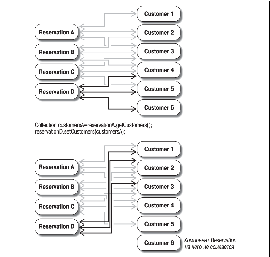
Рис. 7.18. Совместное использование всей коллекции в двунаправленном отношении «многие-ко-многим»
