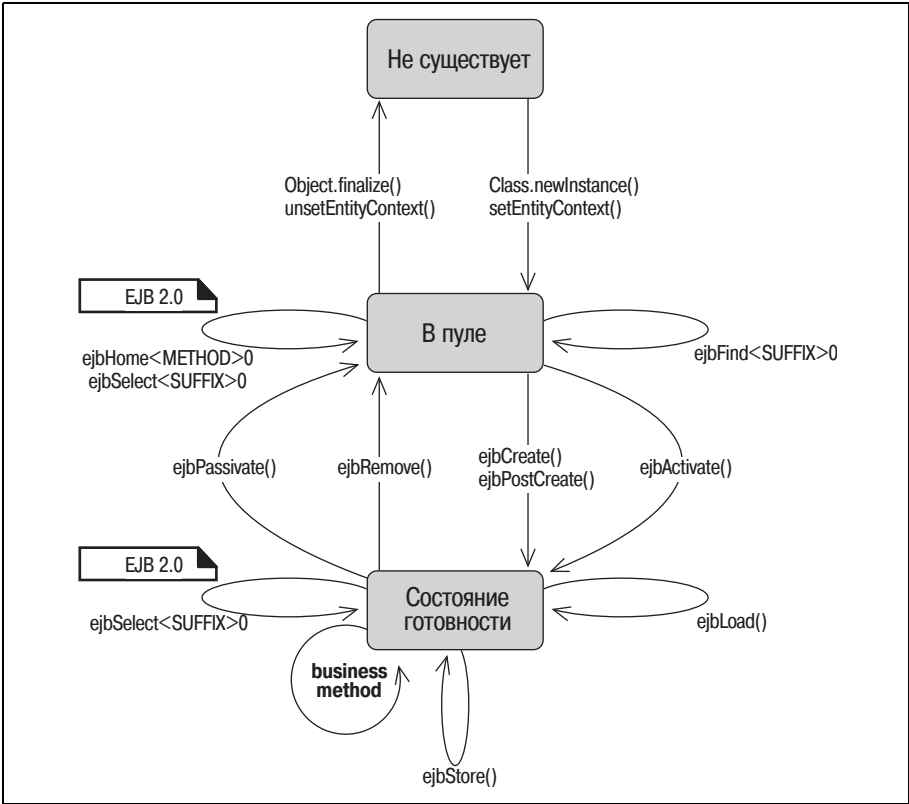
Рис. В.1. Диаграмма состояний жизненного цикла объектного компонента
