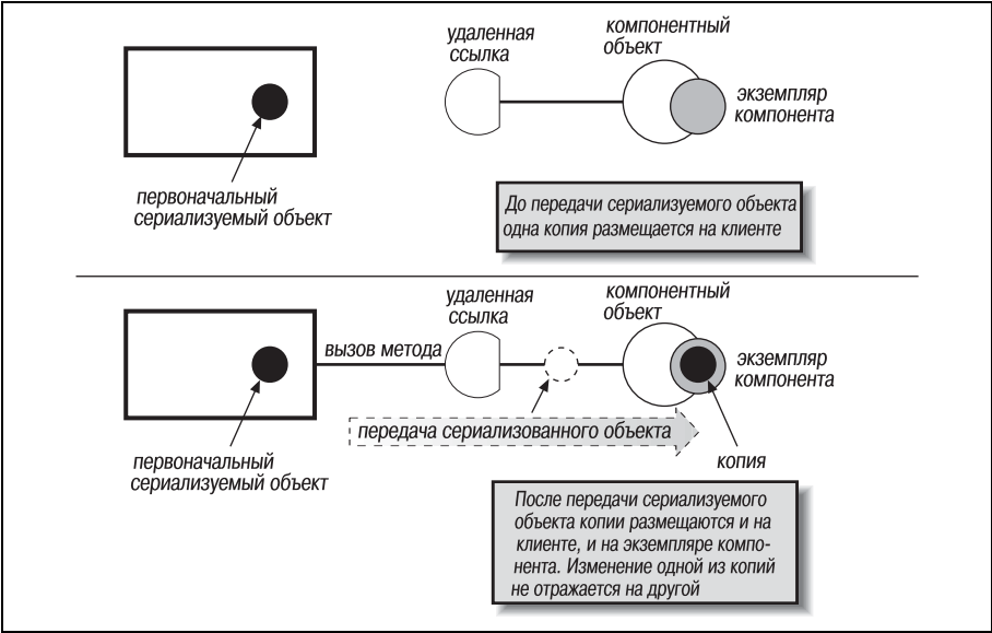
Рис. 5.1. Сериализуемые параметры в Java RMI
