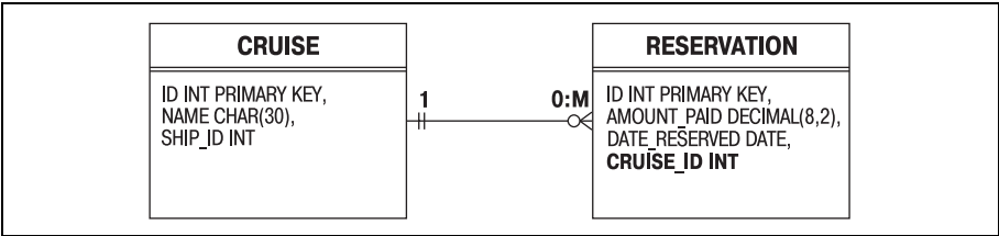
Рис. 7.13. Двухнаправленное отношение «один-ко-многим» / «многие-к-одному» в СУРБД
