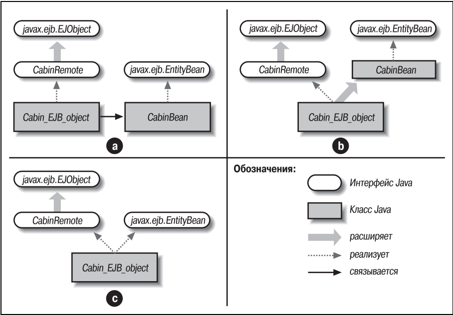
Рис. 2.1. Три способа реализации компонентного объекта
