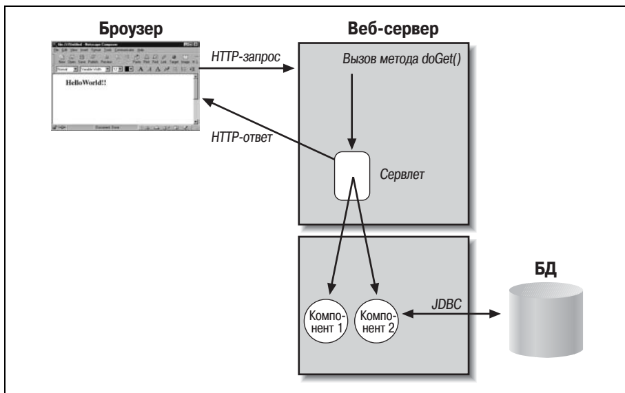
Рис. 17.2. Совместное использование сервлетов/JSP и EJB
