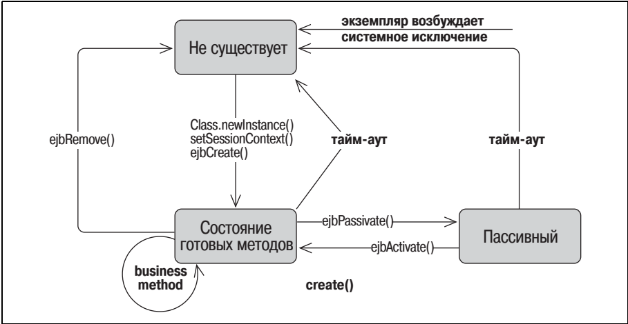
Рис. В.8. Диаграмма состояний жизненного цикла сеансового компонента с состоянием
