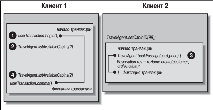
Рис. 14.10. Фантомное чтение
