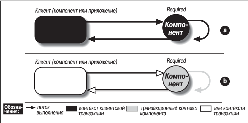
Рис. 14.3. Атрибут Required
