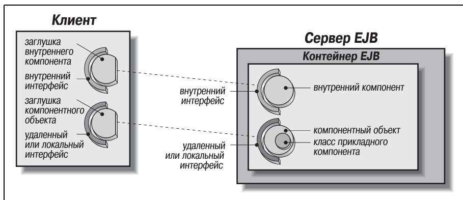
Рис. 2.2. Архитектура EJB
