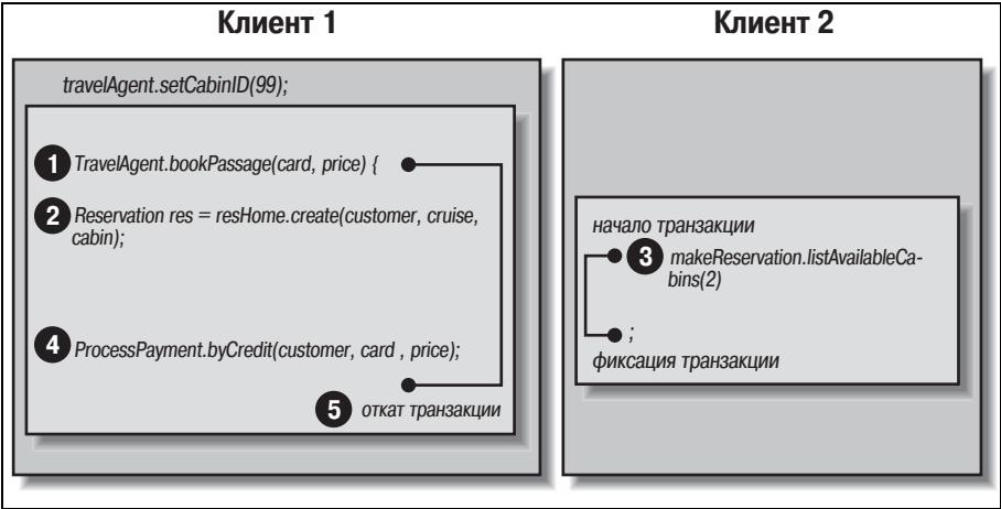
Рис. 14.8. Грязное чтение
