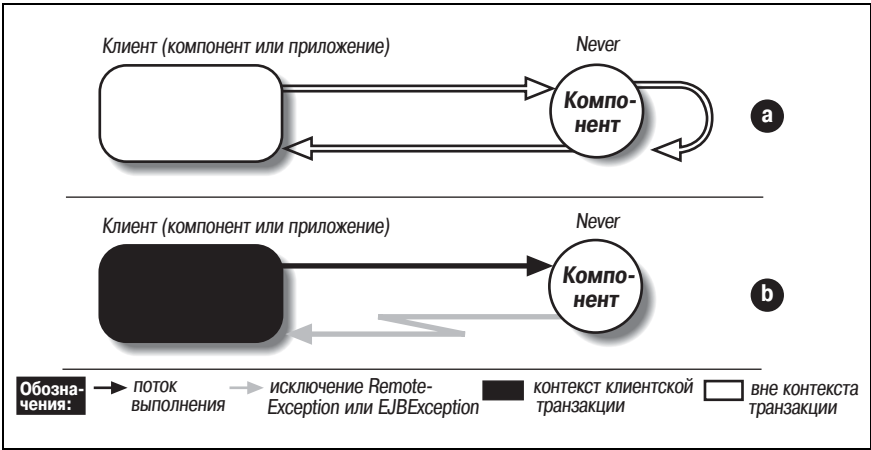
Рис. 14.6. Амрибум Never
