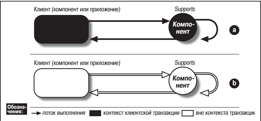
Рис. 14.2. Атрибут Supports
