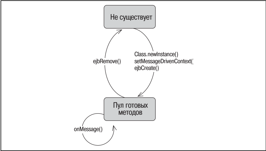
Рис. В.13. Диаграмма состояний жизненного цикла компонента, управляемого сообщениями
