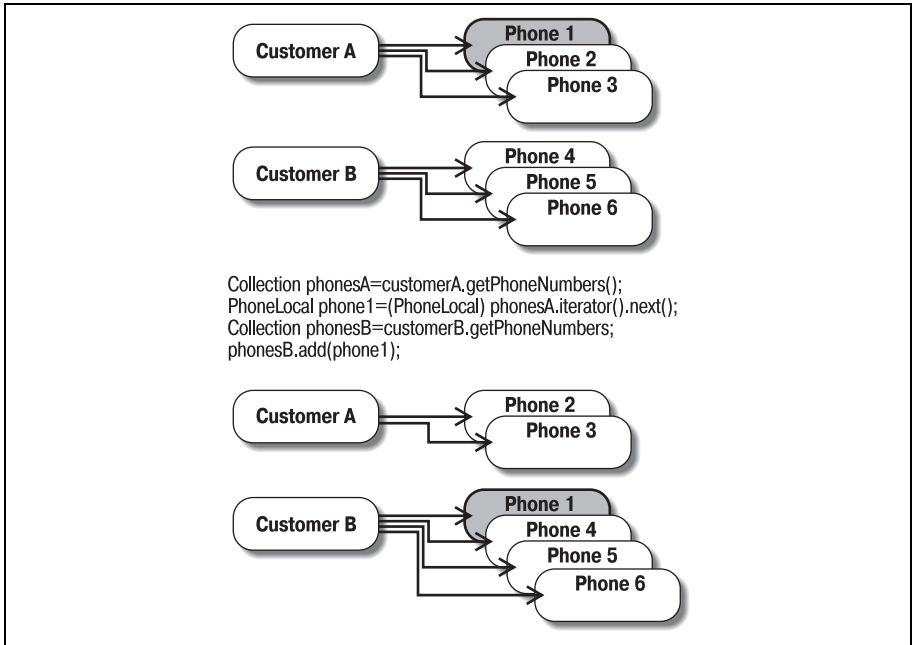
Рис. 7.9. Обмен компонентом в однонаправленном отношении «один-ко-многим»
