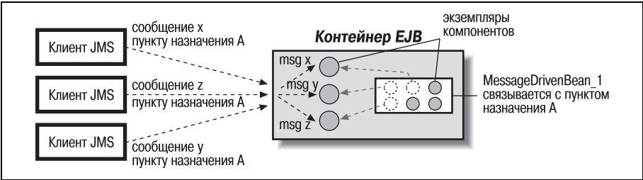
Рис. 3.9. Параллельная обработка в компонентах, управляемых сообщениями
