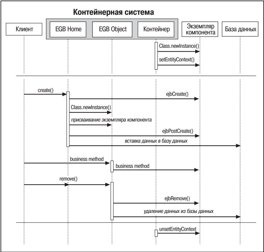
Рис. В.2. Процессы создания и удаления в постоянстве, управляемом контейнером
