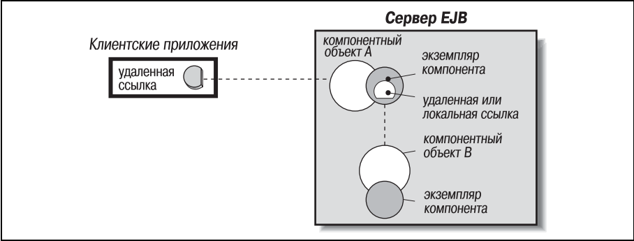
Рис. 3.7. Компоненты обращаются друг к другу через компонентные объекты
