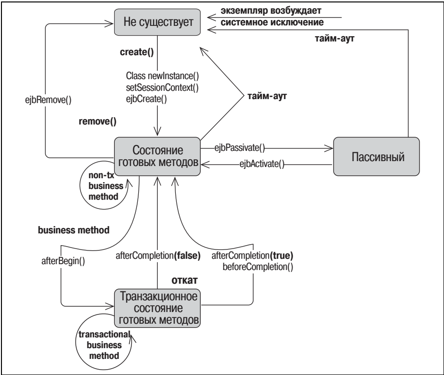
Рис. В.9. Жизненный цикл сеансового компонента с состоянием, использующего интерфейс SessionSynchronization
