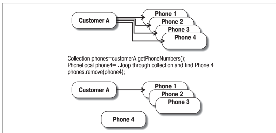
Рис. 7.7. Удаление ссылки на компонент из поля отношения типа «коллекция»
