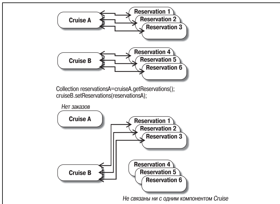
Рис. 7.14. Совместное использование всей коллекции в двунаправленном отношении «один-ко-многим»
