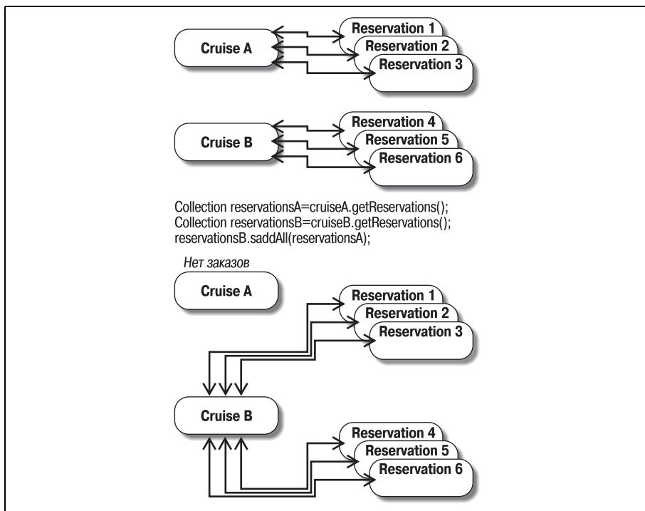
Рис. 7.15. Использование Collection.addAll() в двунаправленном отношении «один-ко-многим»
