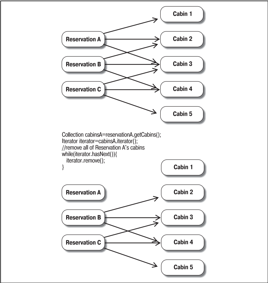
Рис. 7.20. Удаление компонентов в однонаправленном отношении «многие-ко-многим»
