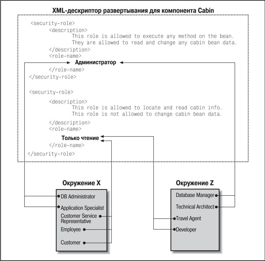
Рис. 3.14. Сопоставление ролей операционного окружения с логическими ролями дескриптора развертывания
