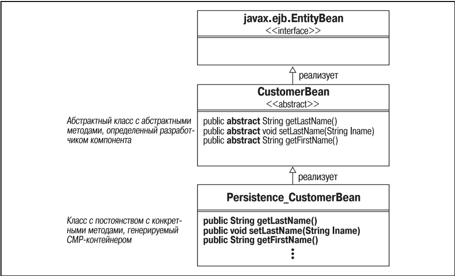
Рис. 6.4. Инструмент контейнера обычно расширяет класс компонента
