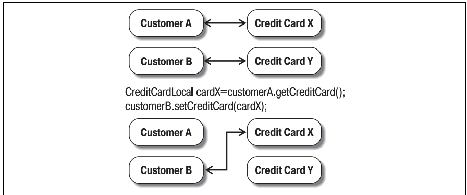
Рис. 7.5. Обмен ссылками в двунаправленных отношениях «один-к-одному»
