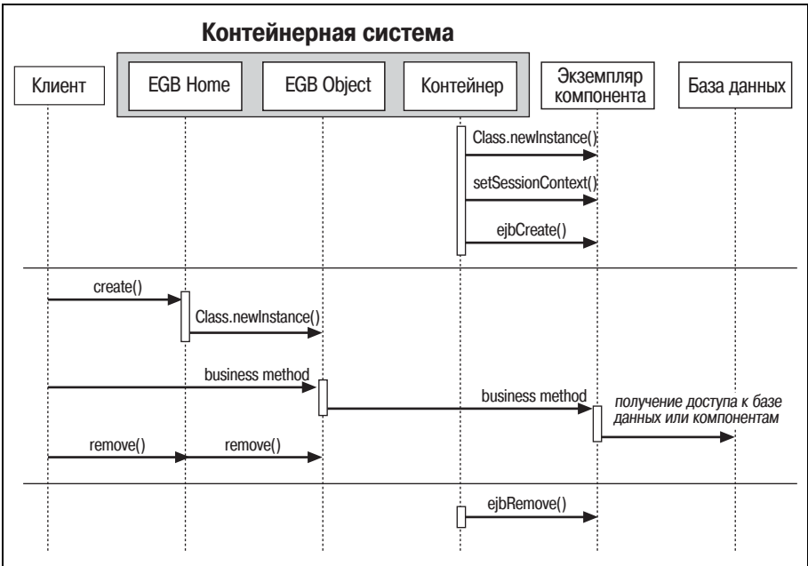
Рис. В.7. Процессы создания и удаления сеансового компонента без состояния
