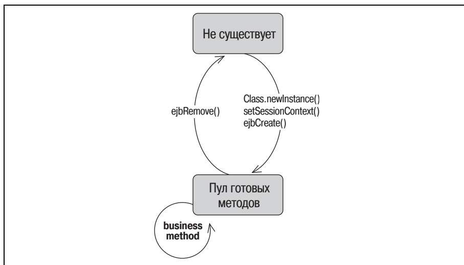
Рис. 12.1. Жизненный цикл сеансового компонента без состояния
