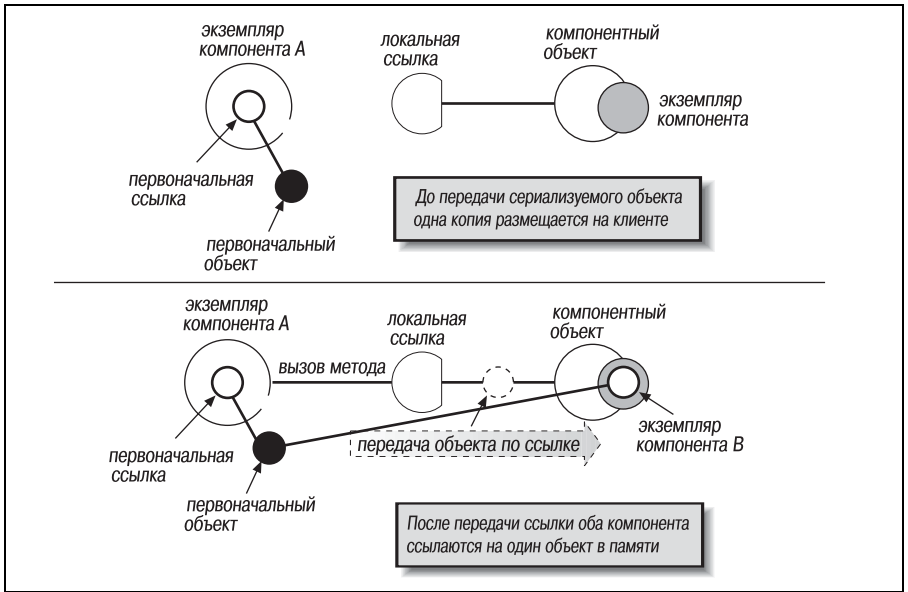
Рис. 5.5. Передача по ссылке с использованием локального клиентского интерфейса
