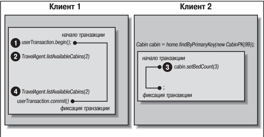
Рис. 14.9. Повторяющееся чтение
