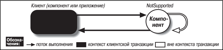
Рис. 14.1. Атрибут NotSupported
