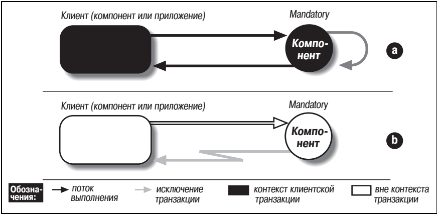
Рис. 14.5. Амрибум Mandatory
