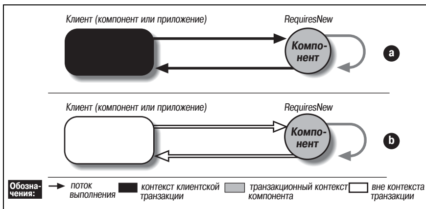
Рис. 14.4. Атрибут RequiresNew
