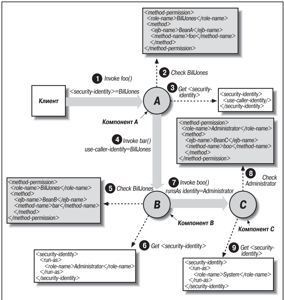
Рис. 3.15. Идентификатор runAs
