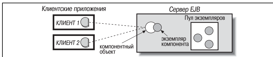
Рис. 3.6. Клиенты, совместно обращающиеся к компонентному объекту
