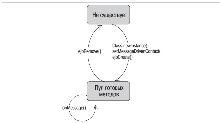
Рис. 13.4. Жизненный цикл MDB
