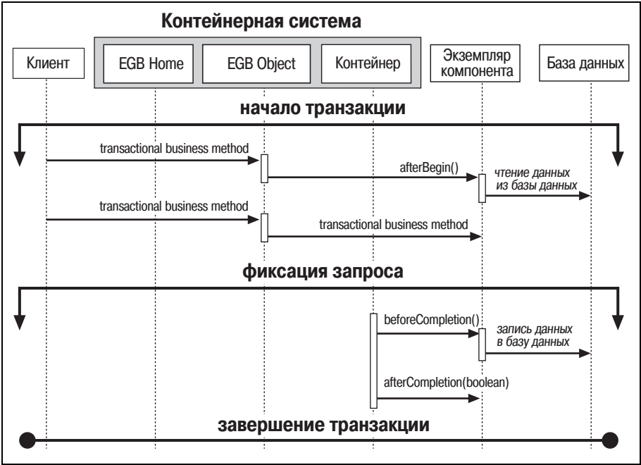
Рис. В.12. Транзакционные уведомления в сеансовых компонентах с интерфейсом SessionSynchronization.
