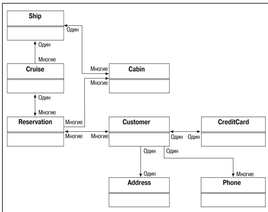
Рис. 7.21. Диаграмма классов «Titan Cruise»
