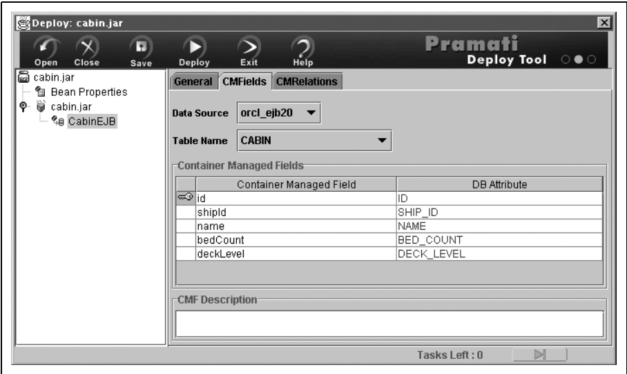
Рис. 3.11. Мастер отображения «объект-отношение» Pramati
