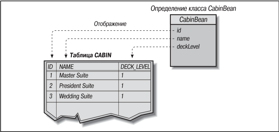
Рис. 3.10. Отображение типа «объект-отношение» объектных компонентов
