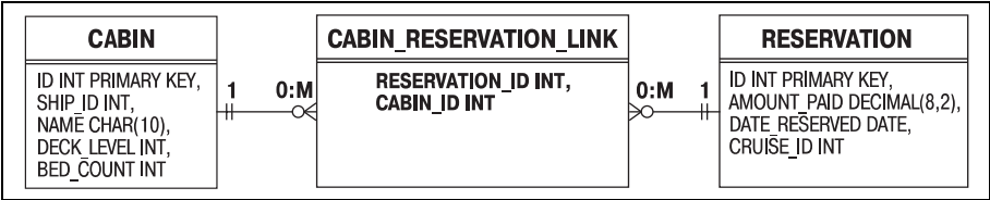
Рис. 7.19. Однонаправленное отношение «многие-ко-многим» в СУРБД
