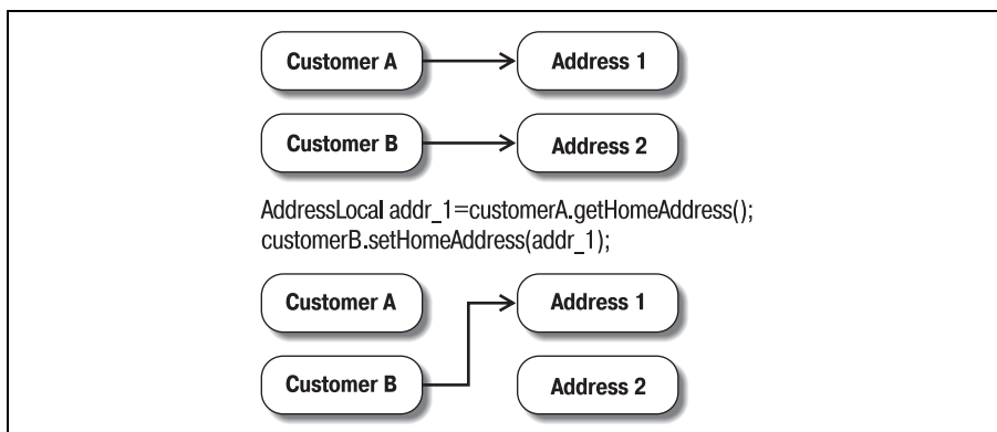
Рис. 7.3. Обмен ссылками в однонаправленных отношениях «один-к-одному»
