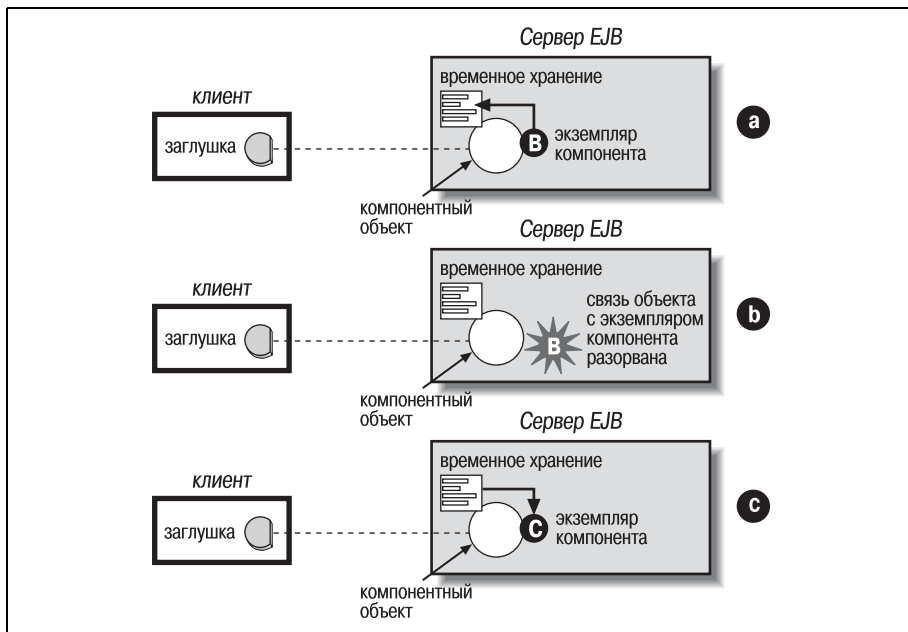
Рис. 3.5. Процессы пассивации и активации
