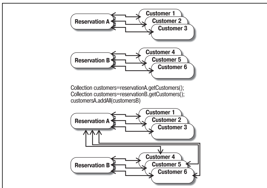
Рис. 7.17. Использование метода Collection.addAll() в двунаправленном отношении «многие-ко-многим»
