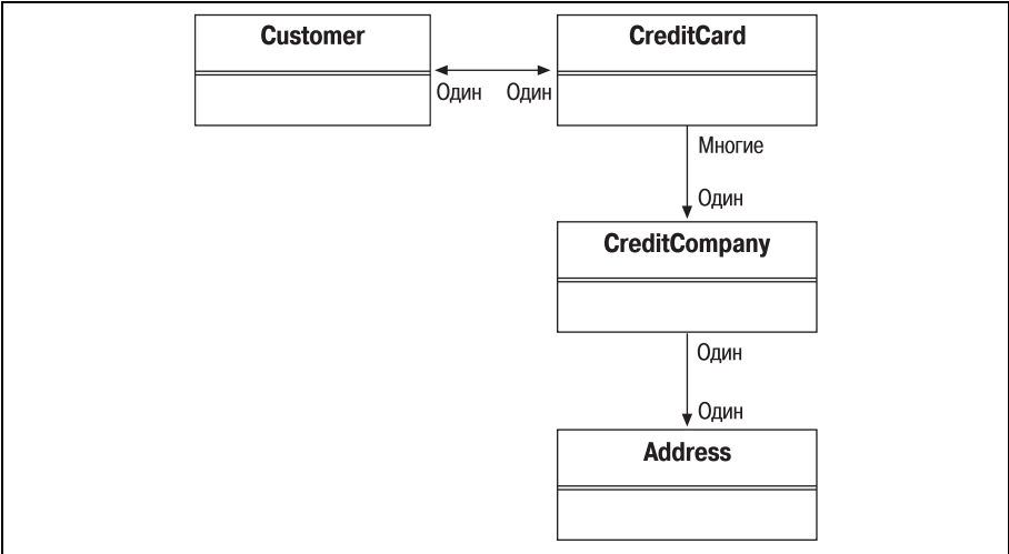
Рис. 8.2. Расширенная диаграмма класса компонента CreditCard
