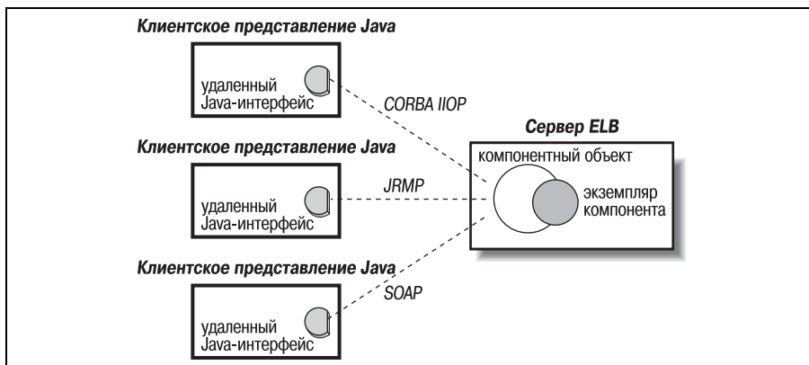
Рис. 3.12. Клиентское представление Java EJB, поддерживаемое различными протоколами
