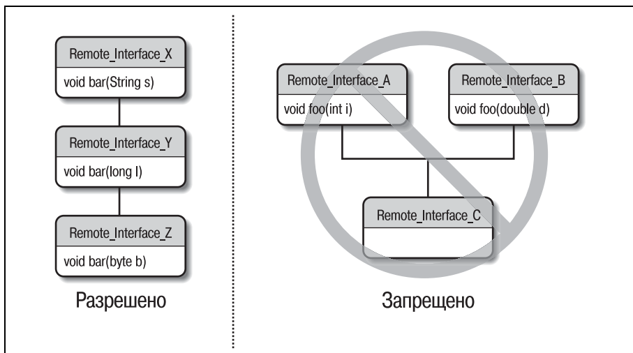
Рис. 5.3. Правила перегрузки при наследовании удаленных интерфейсов в Java RMI-IIOP
