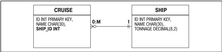
Рис. 7.11. Однонаправленное отношение «многие-к-одному» в СУРБД
