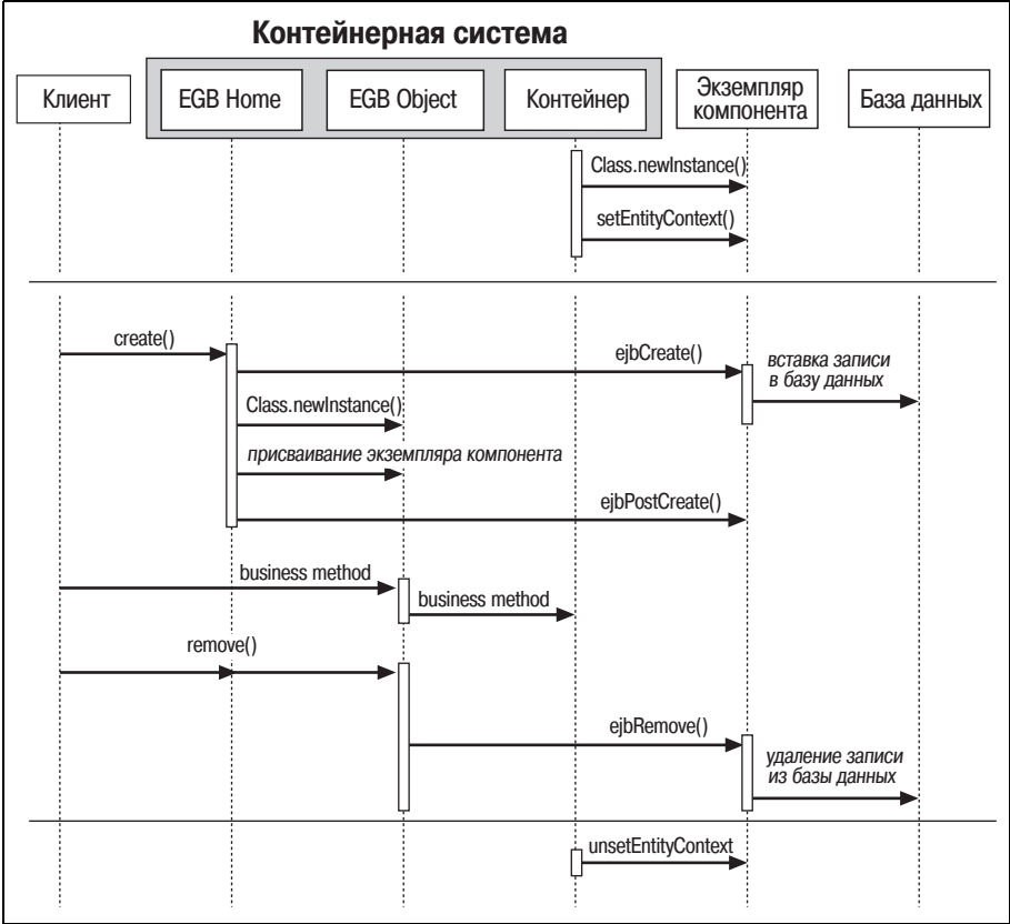
Рис. В.4. Процессы создания и удаления в постоянстве, управляемом компонентом
