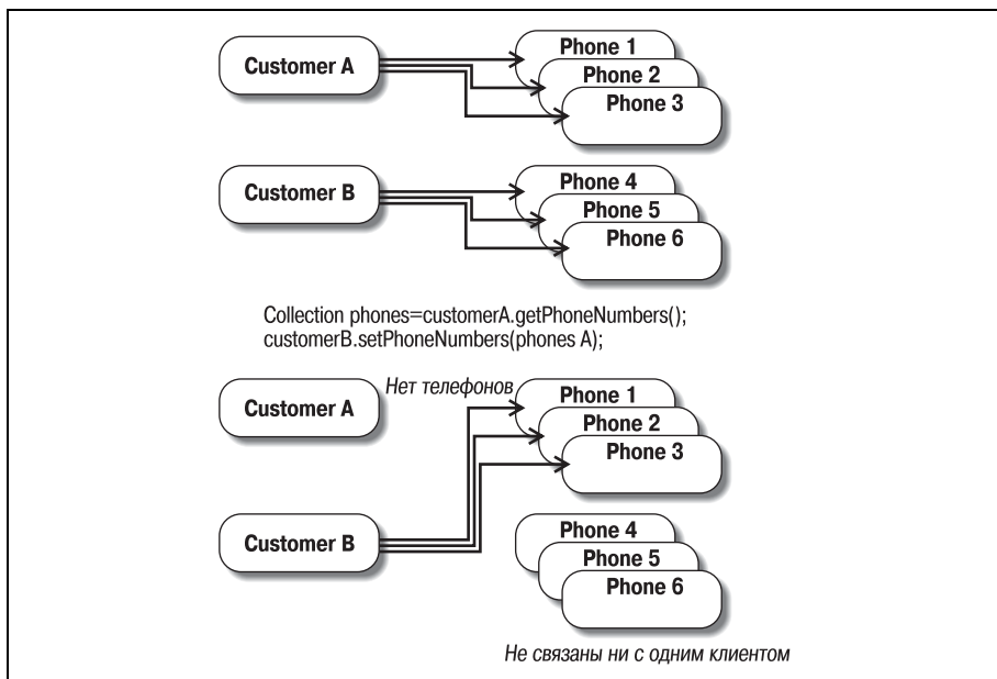
Рис. 7.8. Обмен коллекциями отношений в однонаправленном отношении «один-ко-многим»
