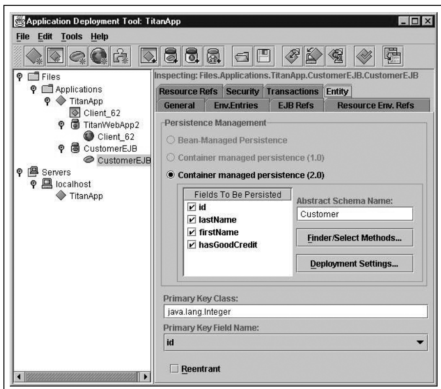
Рис. 6.3. Средство развертывания J2EE 1.3 SDK
