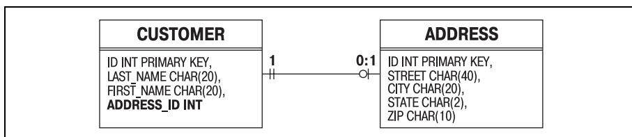
Рис. 7.2. Однонаправленное отношение в СУРБД
