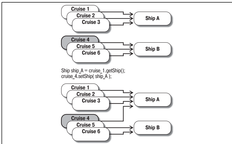
Рис. 7.12. Совместное использование ссылки на компонент в однонаправленном отношении «многие-к-одному»
