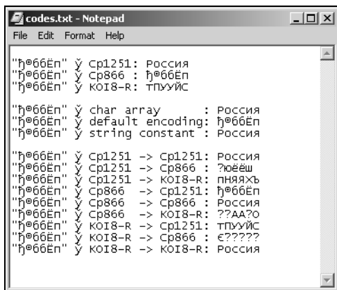
Рис. 5.2. Вывод кириллической строки в файл
