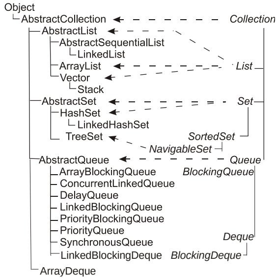
Рис. 6.3. Иерархия классов и интерфейсов-коллекций
