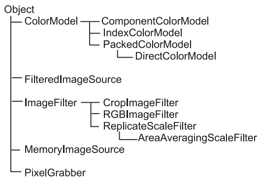
Рис. 20.2. Классы, реализующие модель "поставщик-потребитель"
