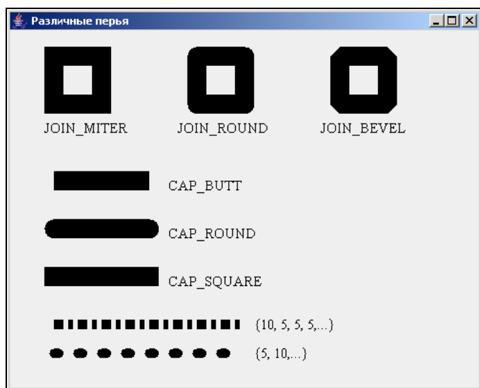
Рис. 9.4. Перья с различными характеристиками
