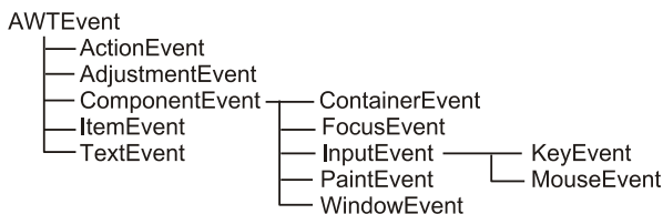
Рис. 15.1. Иерархия классов, описывающих события AWT
