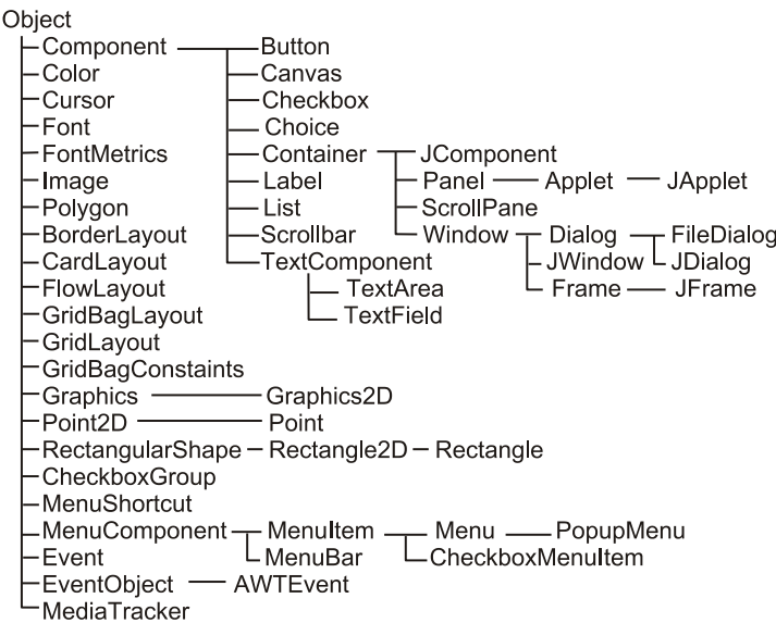
Рис. 8.2. Иерархия основных классов AWT
