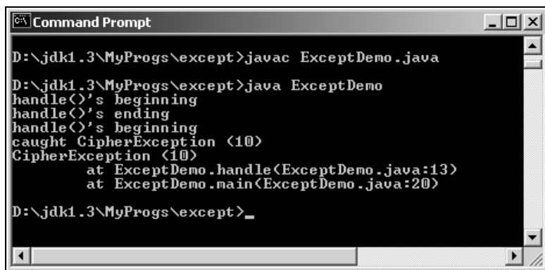
Рис. 21.5. Обработка собственного исключения
