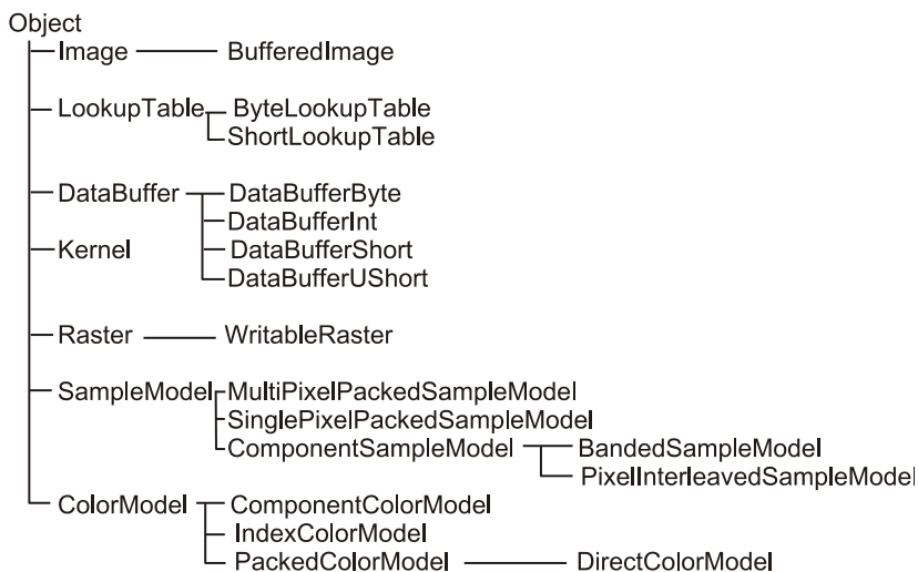
Рис. 20.5. Классы, реализующие модель прямого доступа
