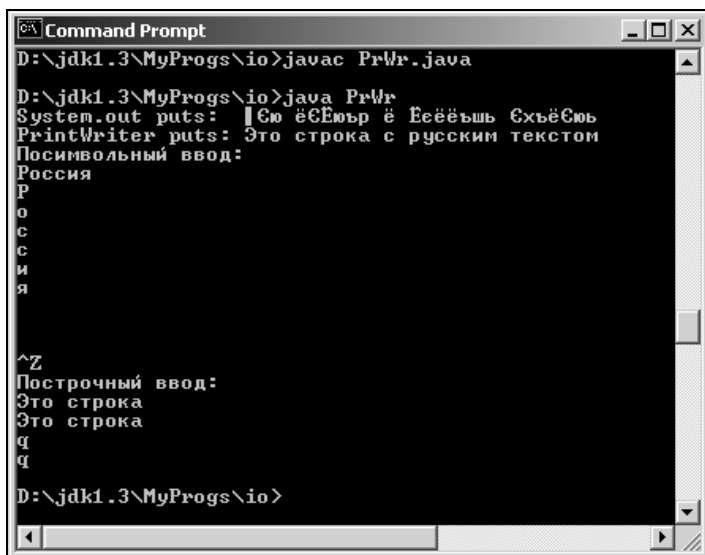
Рис. 23.3. Консольный ввод/вывод
