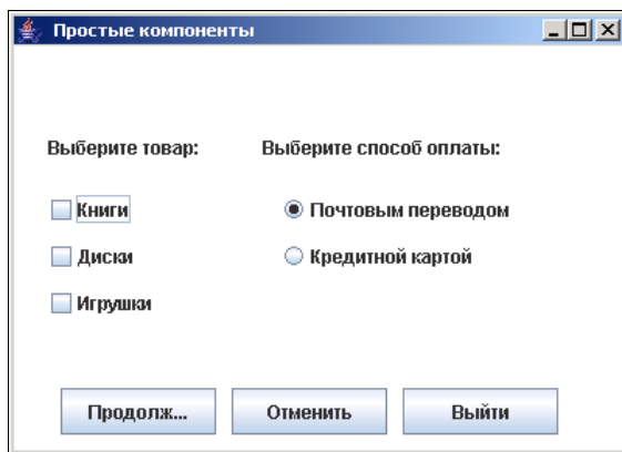
Рис. 10.1. Простые компоненты
