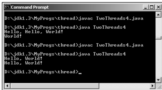
Рис. 22.3. Синхронизация метода
