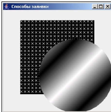
Рис. 9.5. Способы заливки
