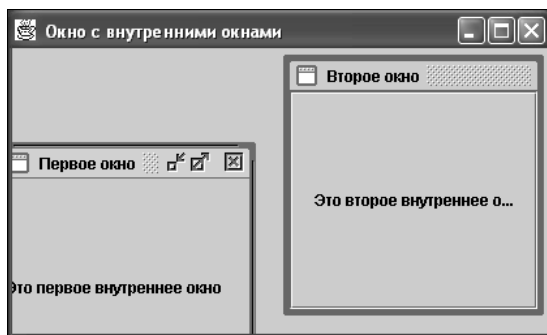
Рис. 14.11. Внутренние окна
