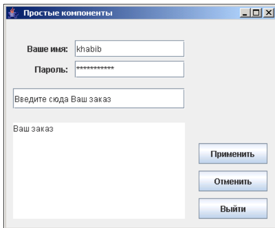
Рис. 10.3. Поля ввода
