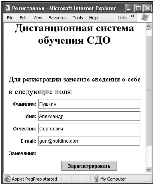
Рис. 26.2. Страница регистрации
