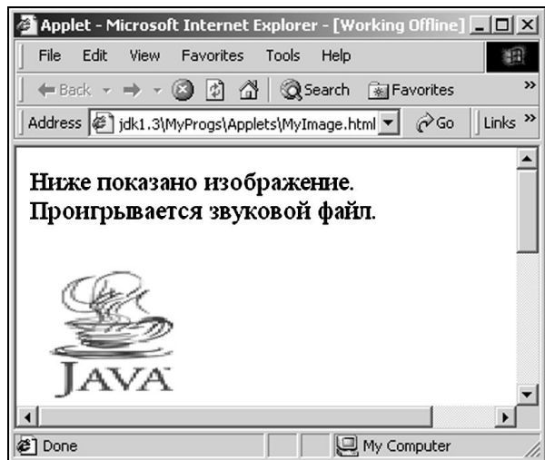
Рис. 18.5. Вывод изображения
