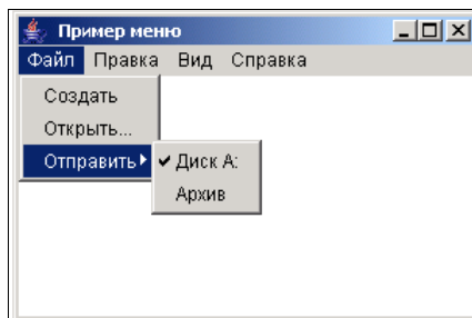
Рис. 10.9. Система меню
