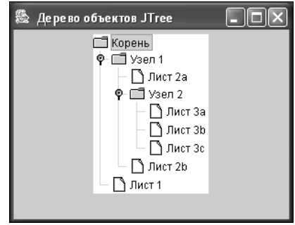
Рис. 11.4. Дерево класса JTree
