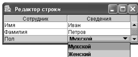
Рис. 13.3. Компонент JComboBox в ячейке таблицы
