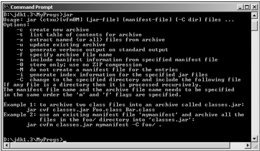
Рис. 25.1. Правила употребления утилиты jar
