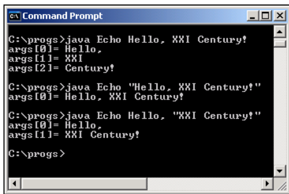
Рис. 2.4. Вывод параметров командной строки
