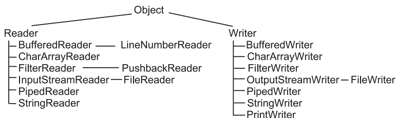
Рис. 23.1. Иерархия классов символьных потоков
