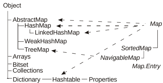
Рис. 6.4. Иерархия классов и интерфейсов-отображений
