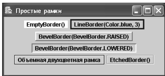
Рис. 16.1. Простые рамки
