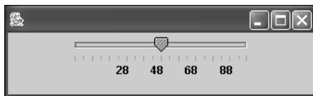
Рис. 11.3. Ползунок JSlider
