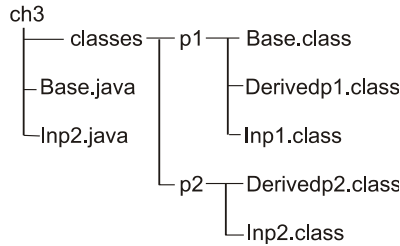
Рис. 3.2. Структура каталогов
