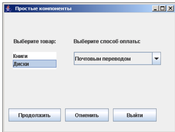
Рис. 10.2. Использование списков
