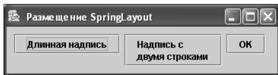
Рис. 14.9. Размещение SpringLayout
