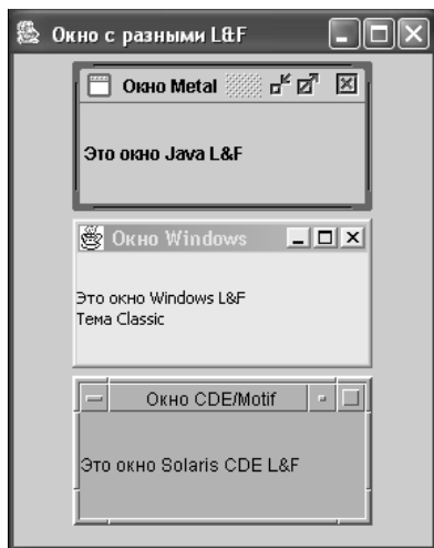
Рис. 17.1. Стандартные L&F
