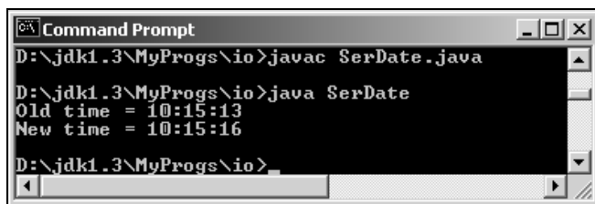
Рис. 23.7. Сериализация объекта
