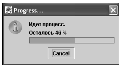
Рис. 14.20. Окно индикатора
