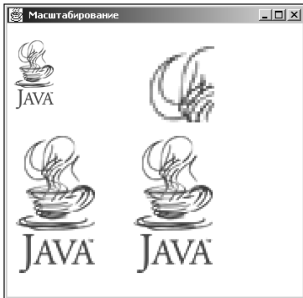
Рис. 20.3. Масштабированное изображение
