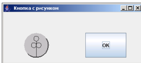
Рис. 10.8. Круглая кнопка
