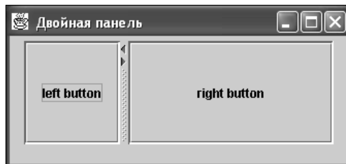
Рис. 14.7. Двойная панель
