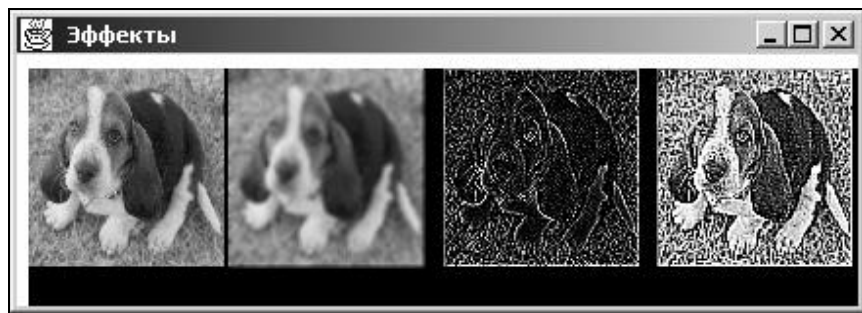
Рис. 20.8. Создание эффектов
