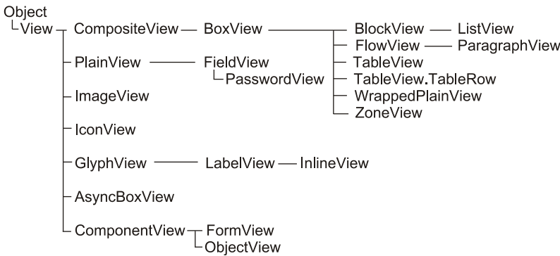
Рис. 12.1. Иерархия классов-видов
