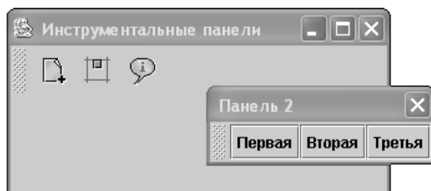
Рис. 14.10. Инструментальные панели
