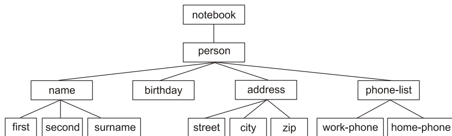
Рис. 28.1. Дерево элементов документа XML
