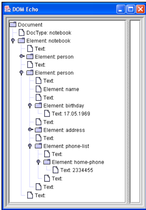
Рис. 28.2. Дерево объектов документа XML
