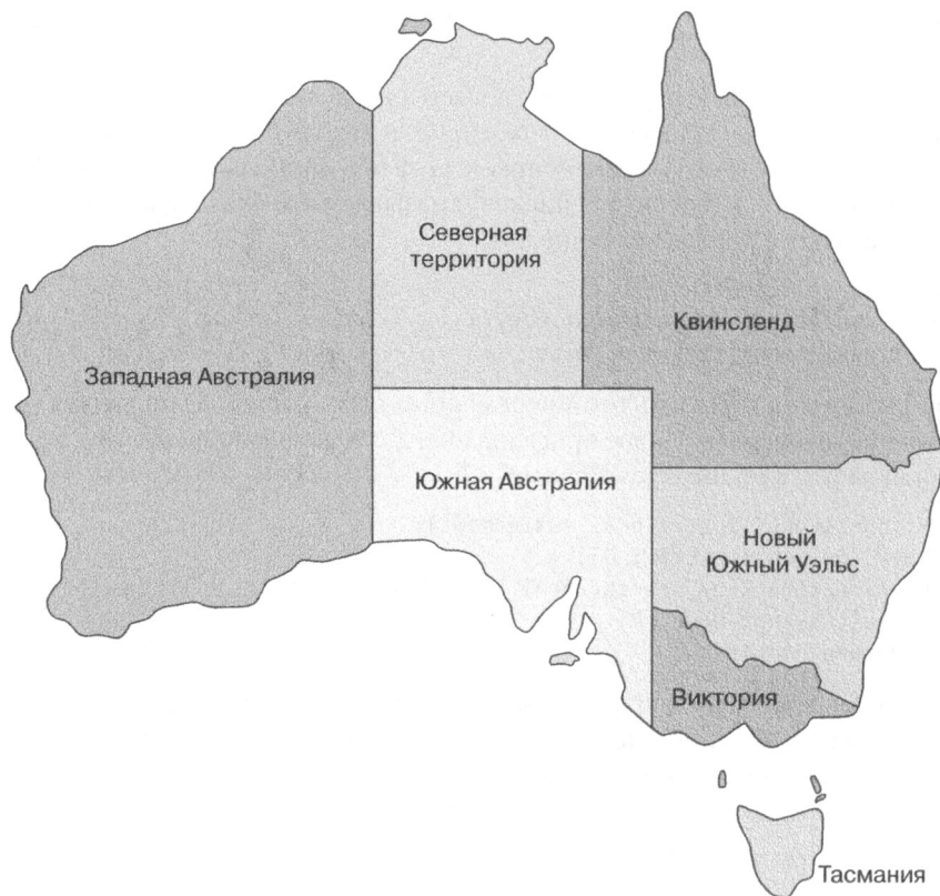
Рис. 3.2. В решении задачи раскраски карты Австралии никакие две смежные ее части не могут быть окрашены в один и тот же цвет
