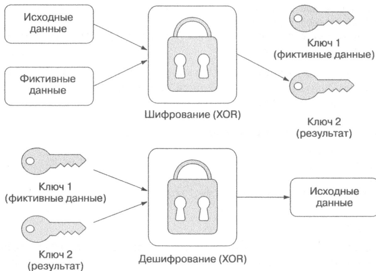
Рис. 1.6. Одноразовый шифр приводит к созданию двух ключей, которые можно разделить, а затем объединить для восстановления исходных данных
