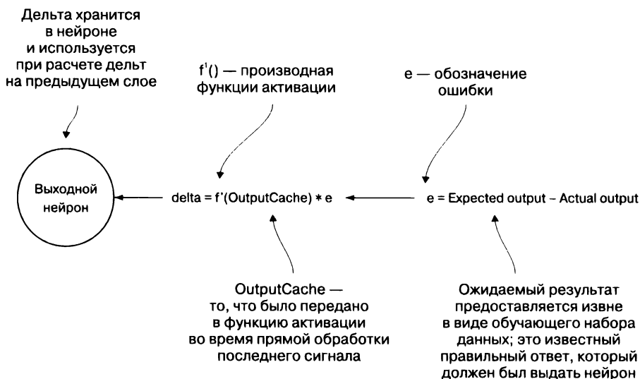
Рис. 7.4. Механизм, с помощью которого вычисляется дельта выходного нейрона на этапе обучения посредством обратного распространения
