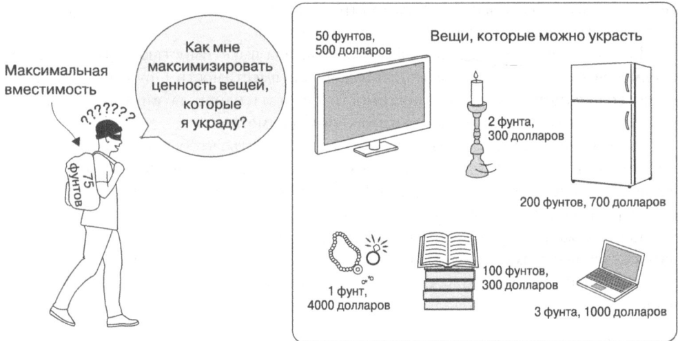
Рис. 9.1. Взломщику необходимо решить, какие предметы украсть, потому что вместимость рюкзака ограничена
