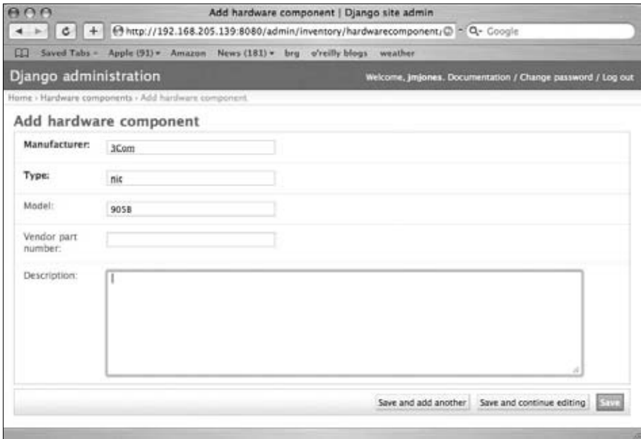
Рис. 11.9. Форма добавления аппаратного компонента в административном интерфейсе Django
