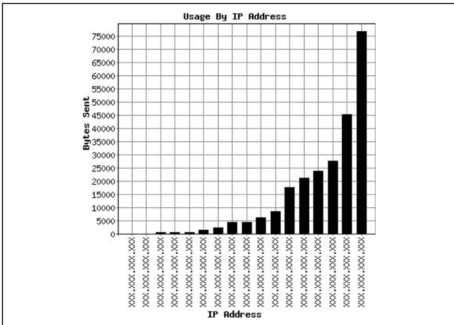
Рис. 4.1. Гистограмма количества байтов, переданных по запросам с каждого IP-адреса
