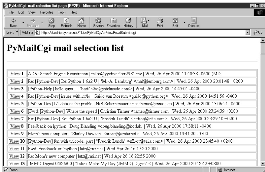
Рис. 13.8. Страница списка выбора сообщений PyMailCgi , верх
