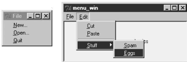
Рис. 8.3. Отрывное меню File и каскадное Edit
