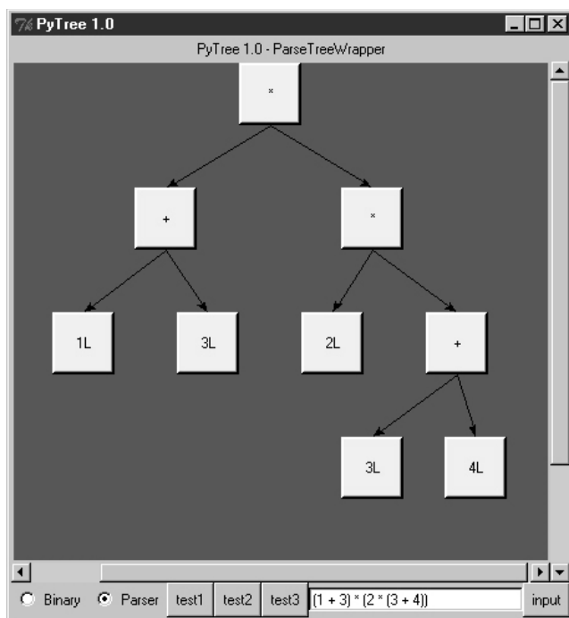
Рис. 18.4. Дерево синтаксического разбора для « (1 + 3) * (2 * (3 + 4)) »
