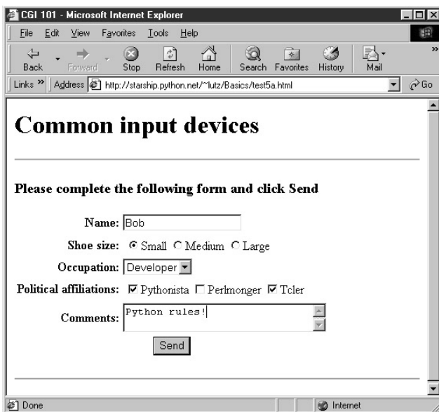
Рис. 12.13. Страница формы, генерируемая test5a.html
