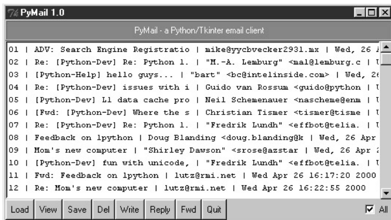
Рис. 13.12. Тот же самый список сообщений в PyMailGui
