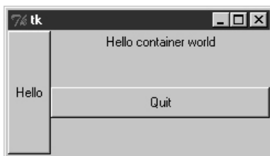
Рис. 6.18. gui4 увеличивается в расширяемом фрейме
