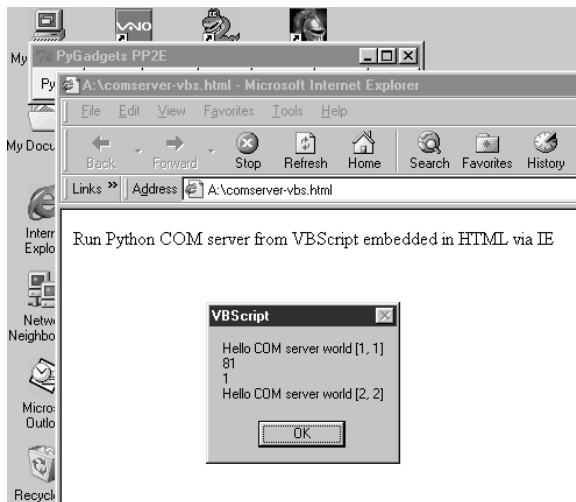
Рис. 15.9. IE, выполняющий клиент VBScript, выполняющий COM-сервер Python
