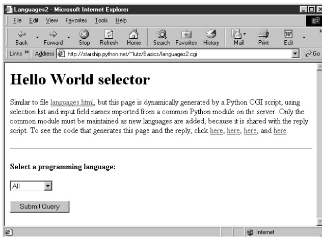
Рис. 12.23. Альтернативная главная страница, созданная languages2.cgi
