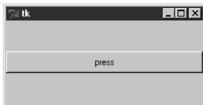
Рис. 6.10. Изменение размера при expand=YES , fill=X
