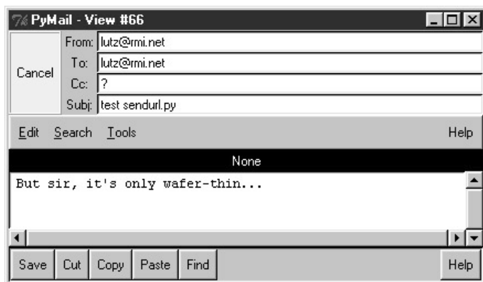
Рис. 13.6. Результат sendurl.py
