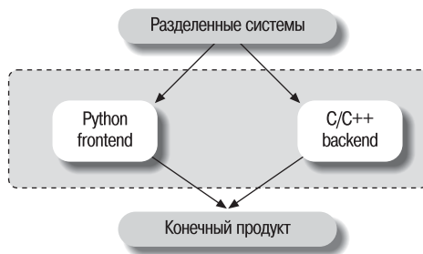
Рис. 21.4. Гибридная архитектура
