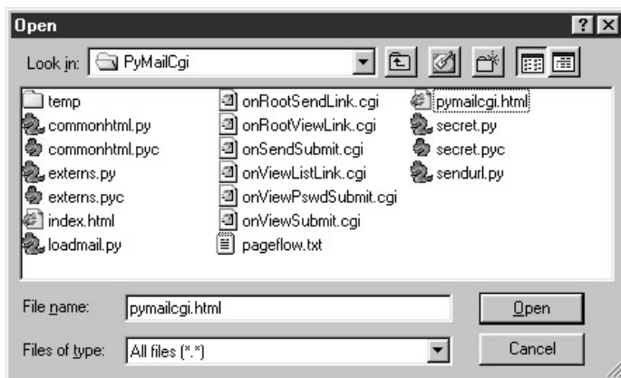
Рис. 13.1. Содержание PyMailCgi
