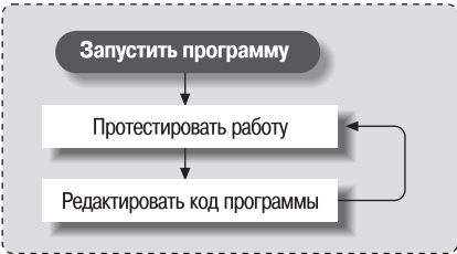
Рис. 21.1. Циклы разработки
