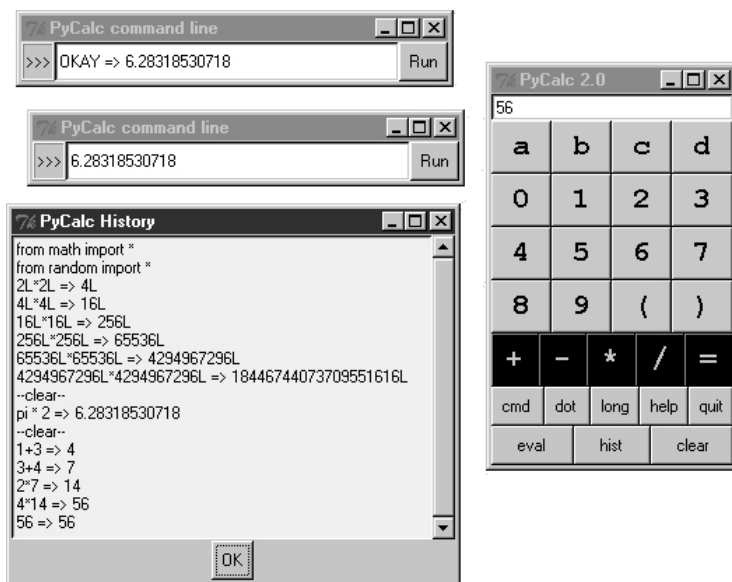
Рис. 18.11. Калькулятор PyCalc с некоторыми всплывающими окнами
