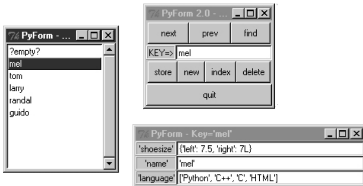
Рис. 16.3. Полка словарей ( dbinit2 , dbview )
