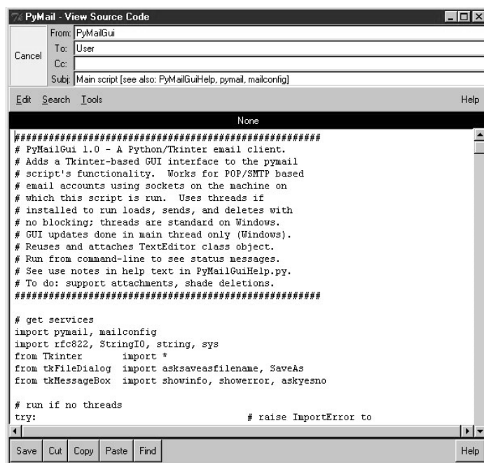
Рис. 11.12. Окно просмотра исходного кода PyMailGui
