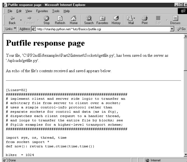
Рис. 12.36. Новый putfile с загруженным getfile , основанным на сокетах
