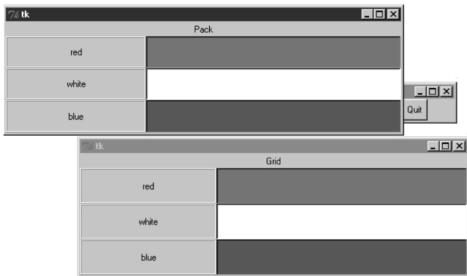
Рис. 8.29. Окна grid и pack после изменения размера
