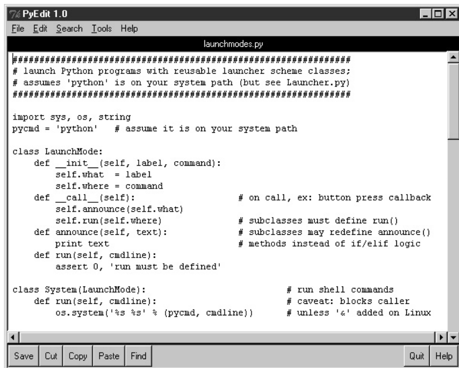
Рис. 3.2. Программа PyEdit, запущенная с помощью launchmodes
