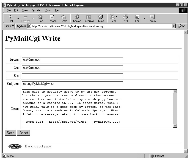
Рис. 13.3. Страница PyMailCgi отправки (составления) сообщения
