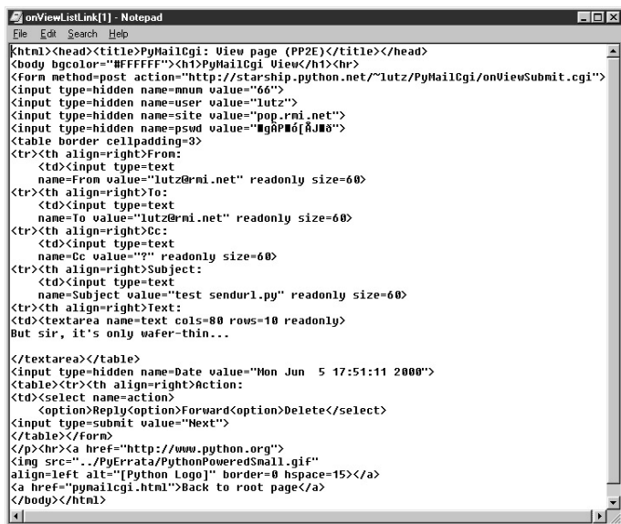
Рис. 13.14. HTML, сгенерированный для страницы просмотра PyMailCgi
