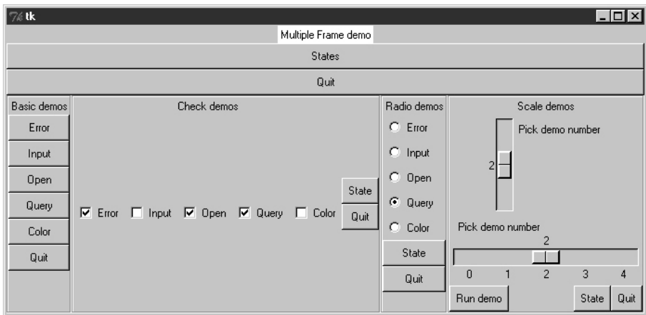
Рис. 7.30. demoAll_frm : вложенные фреймы
