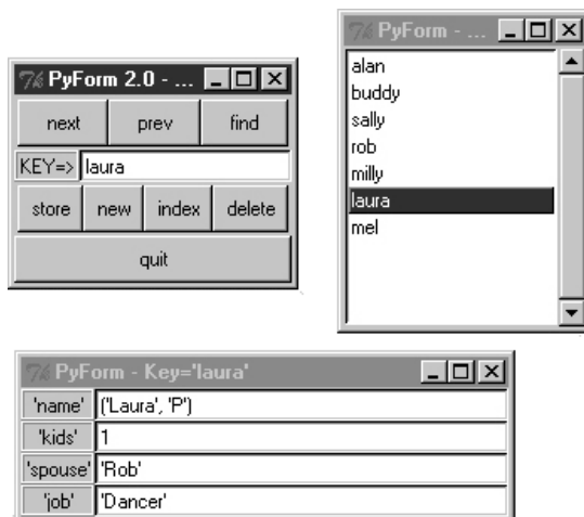
Рис. 16.1. PyForm выводит полку с объектами Actor
