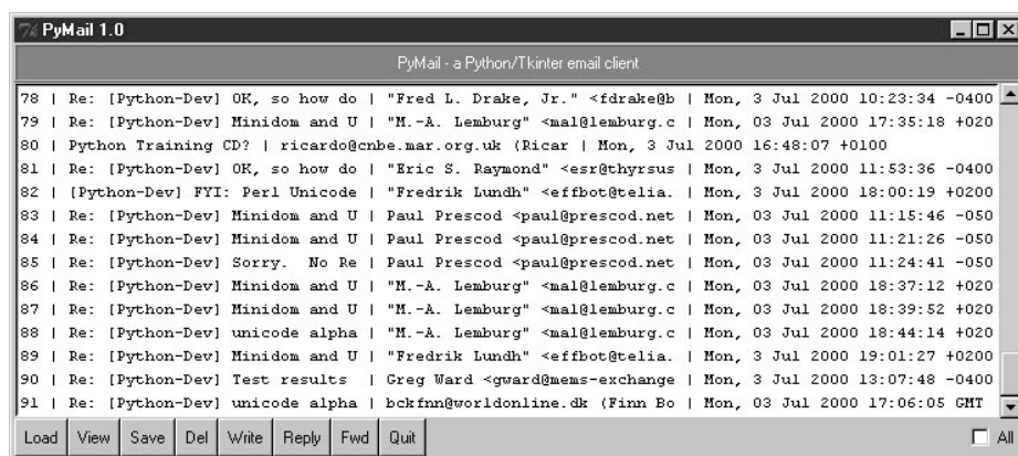
Рис. 11.18. Главное окно PyMailGui с измененными размерами
