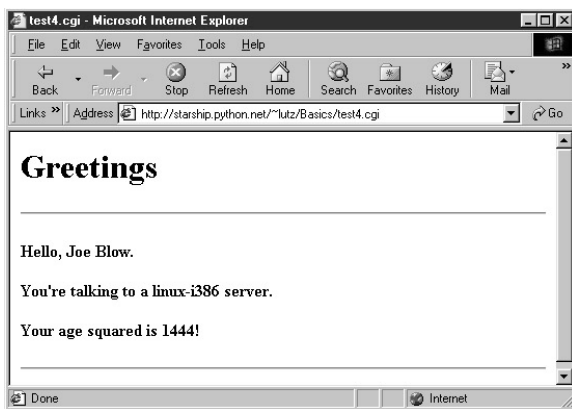
Рис. 12.11. Страница ответа, сгенерированная test4.cgi
