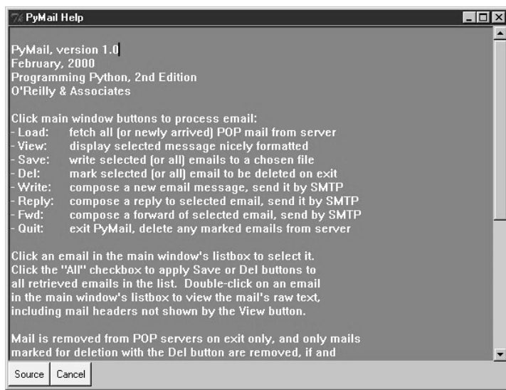
Рис. 11.11. Всплывающее окно подсказки PyMailGui
