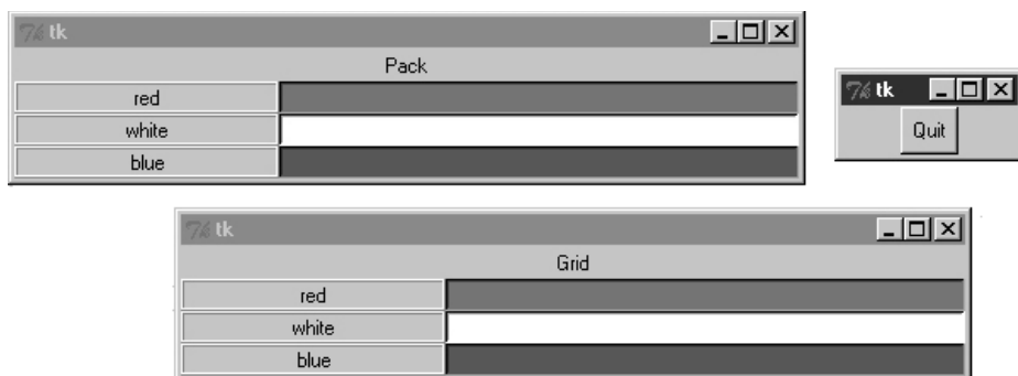
Рис. 8.28. Окна grid и pack до изменения размеров
