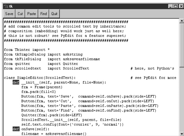
Рис. 8.17. simpleedit в действии
