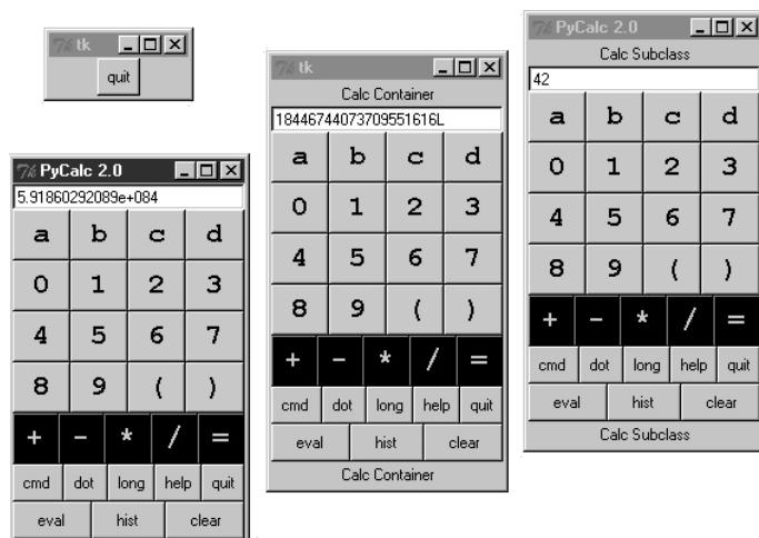
Рис. 18.13. Сценарий calculator_test : прикрепление и расширение
