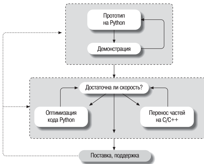
Рис. 21.5. Создание прототипов на Python
