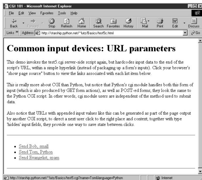
Рис. 12.17. Страница гиперссылок, созданная test5c.html
