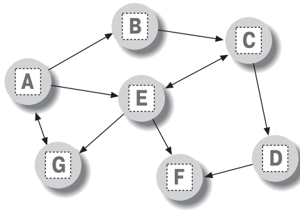
Рис. 17.1. Направленный граф
