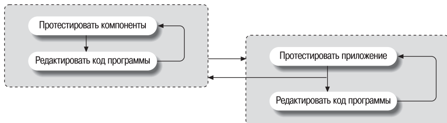
Рис. 21.2. Инкрементная разработка
