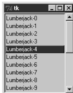
Рис. 8.12. scrolledlist вверх
