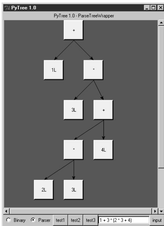
Рис. 18.1. Дерево синтаксического разбора для 1 + 3 * (2 * 3 + 4)
