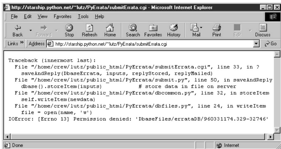
Рис. 14.26. Передача сообщения об ошибке, исключительная ситуация (требуется chmod 777 dir )
