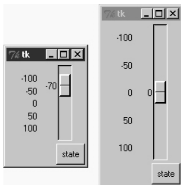
Рис. 7.29. Простая шкала без переменных
