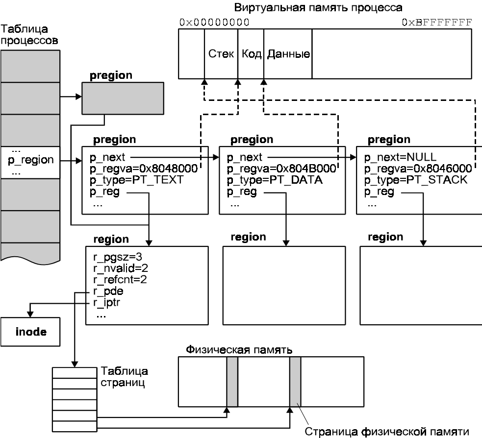
Рис. 3.10. Управление адресным пространством процесса в SCO UNIX
