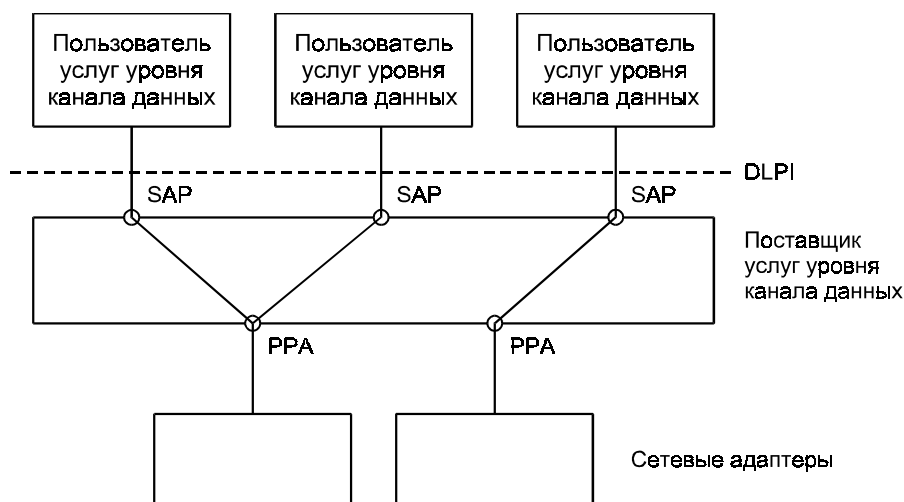
Рис. 6.43. Доступ к услугам поставщика услуг уровня канала данных
