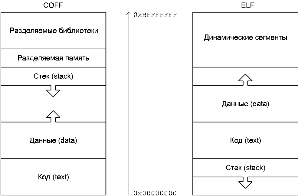
Рис. 3.9. Виртуальная память процесса в режиме задачи
