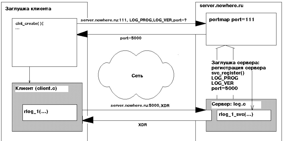
Рис. 6.28. Работа системы RPC
