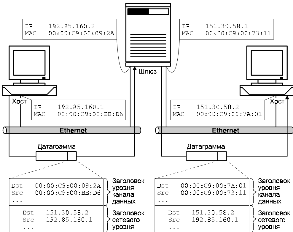
Рис. 6.34. Инкапсуляция пакетов для косвенных маршрутов
