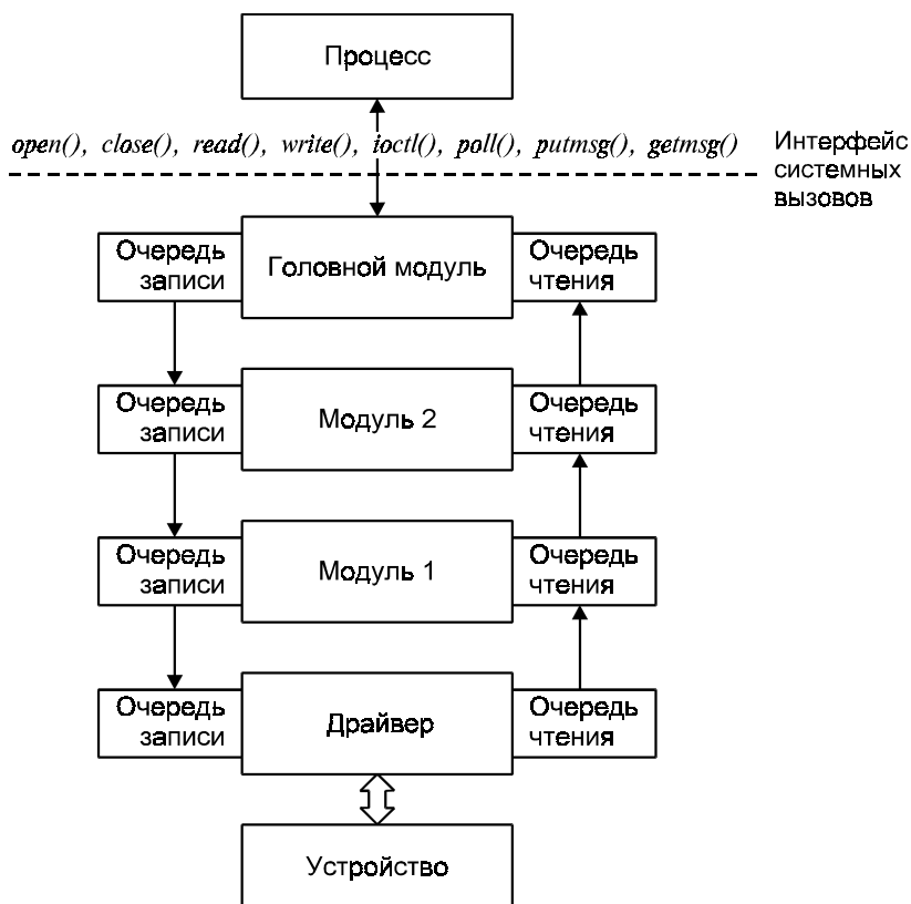
Рис. 5.13. Базовая архитектура потока
