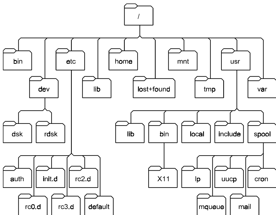
Рис. 1.4. Типичная файловая система UNIX
