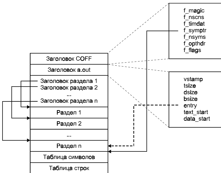
Рис. 2.5. Структура исполняемого файла в формате COFF
