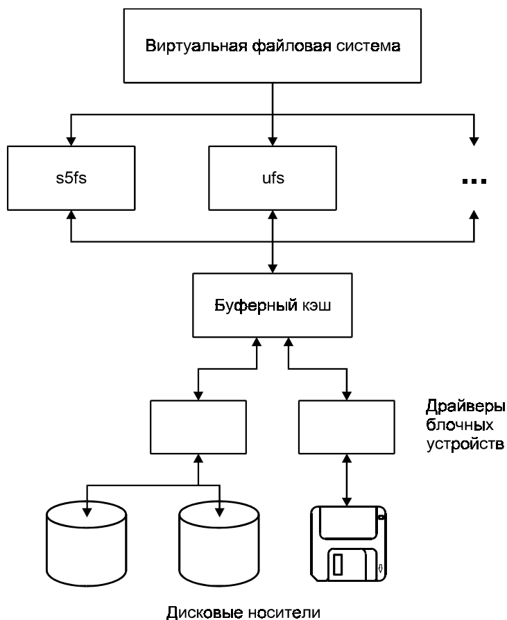
Рис. 4.13. Роль буферного кэша
