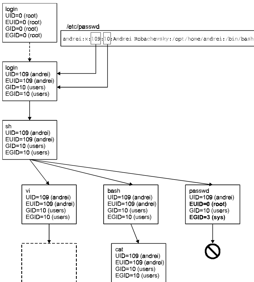
Рис. 2.10. Наследование пользовательских идентификаторов
