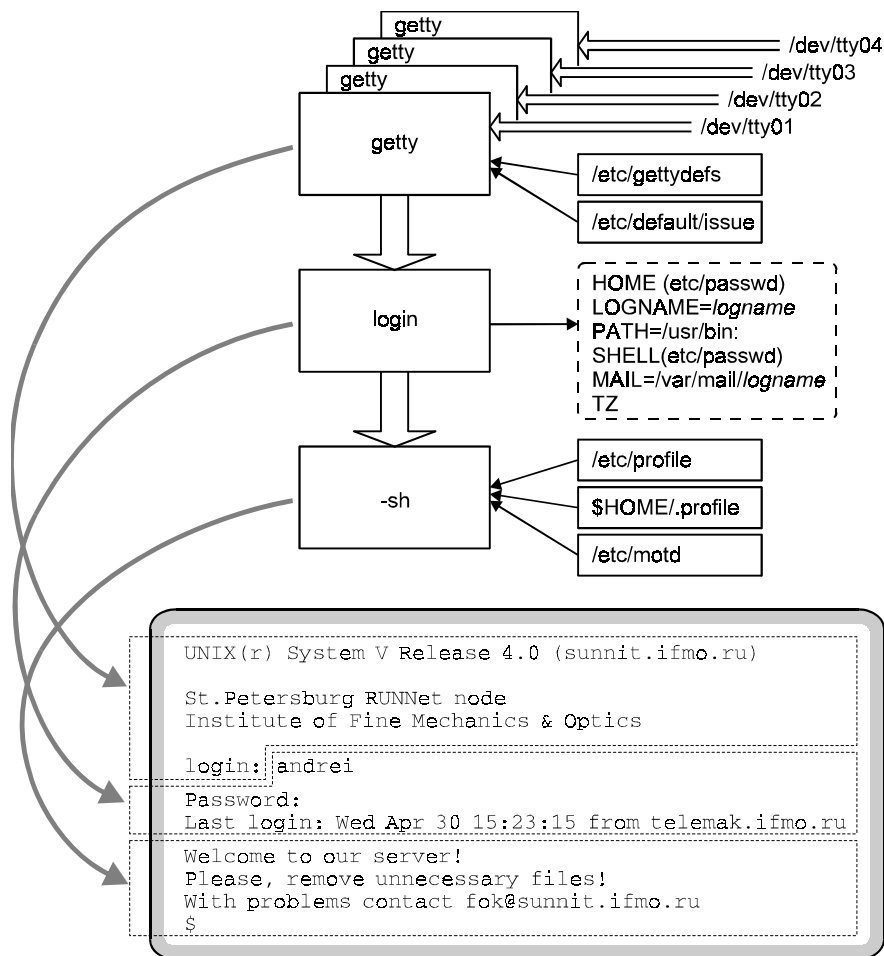
Рис. 1.8. Процессы, обеспечивающие вход пользователя в систему
