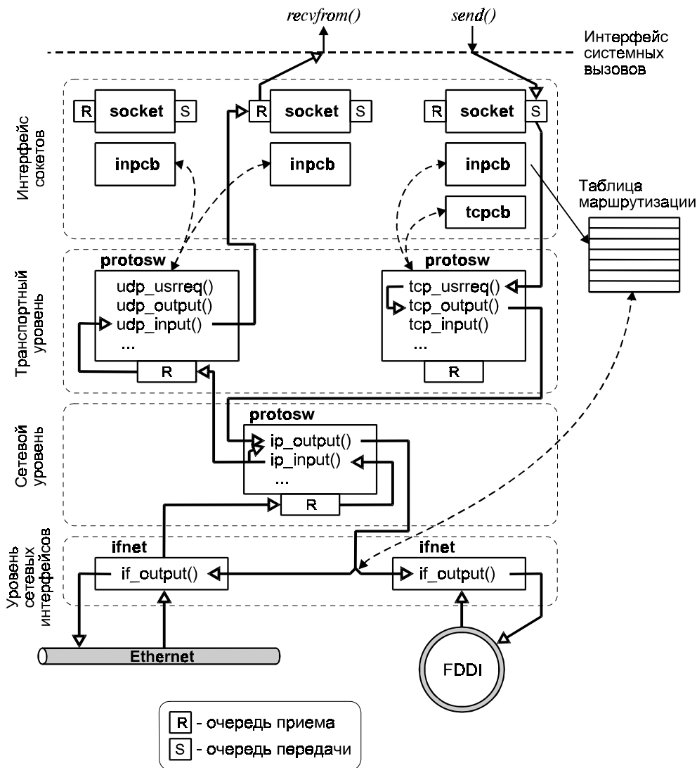
Рис. 6.37. Сетевая подсистема BSD UNIX
