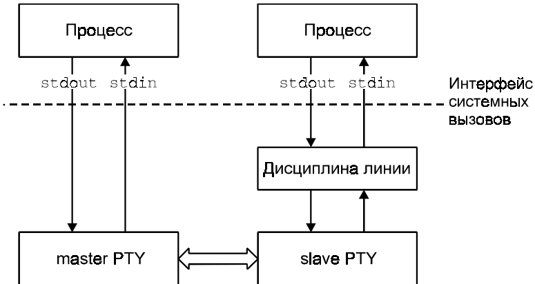
Рис. 5.11. Взаимодействие процессов с помощью псевдотерминала
