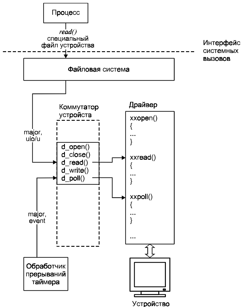
Рис. 5.2. Доступ к драйверу символического устройства
