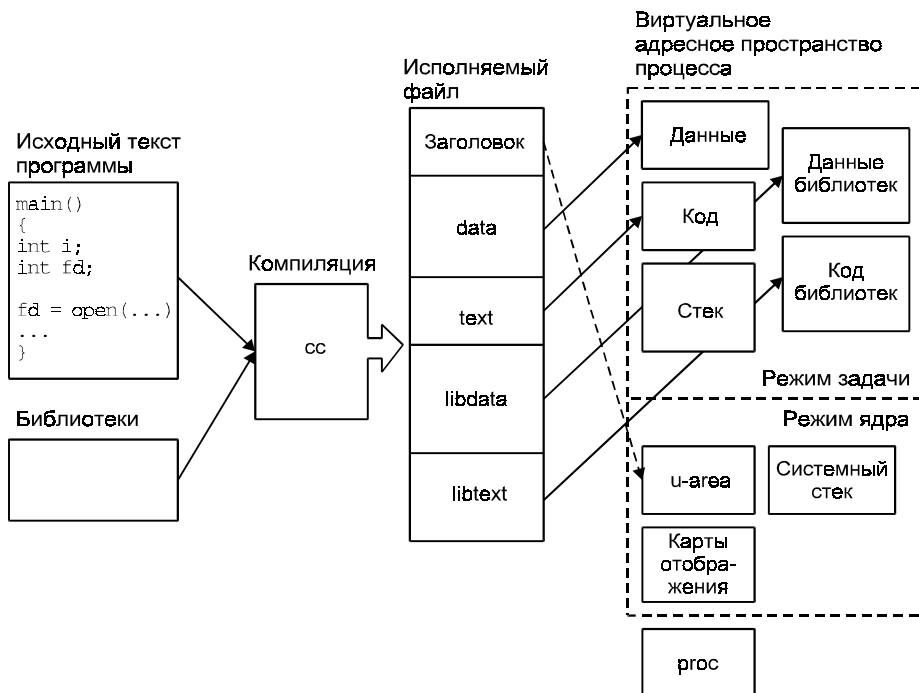
Рис. 3.1. Инфраструктура процесса операционной системы UNIX
