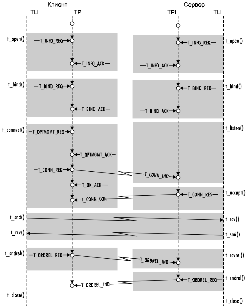
Рис. 6.40. Функции TLI/XTI и примитивы TPI
