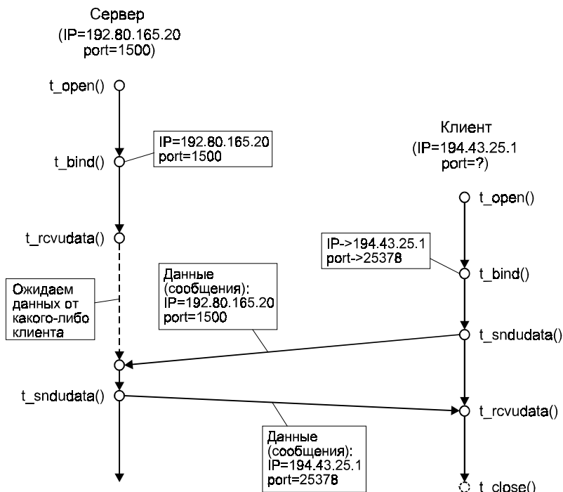
Рис. 6.26. Схема вызова функций TLI/XTI для протокола с предварительным установлением соединения
