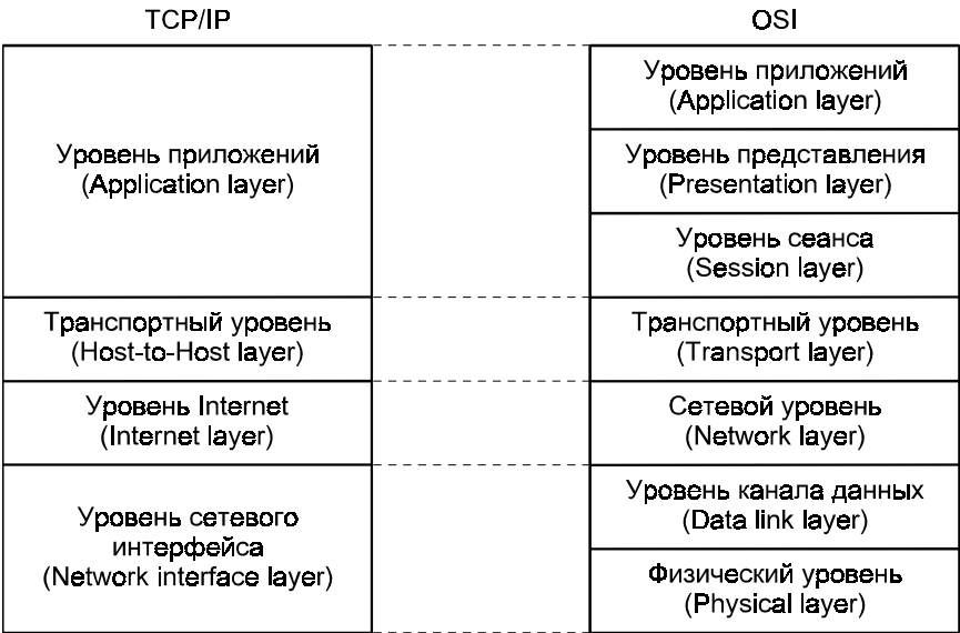
Рис. 6.4. Соответствие между моделями TCP/IP и OSI
