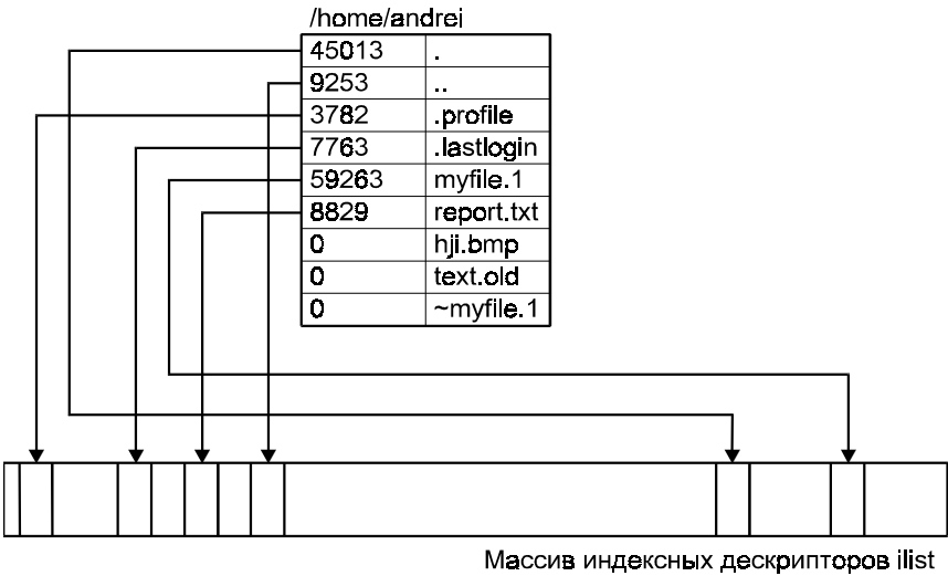
Рис. 4.3. Каталог файловой системы s5fs
