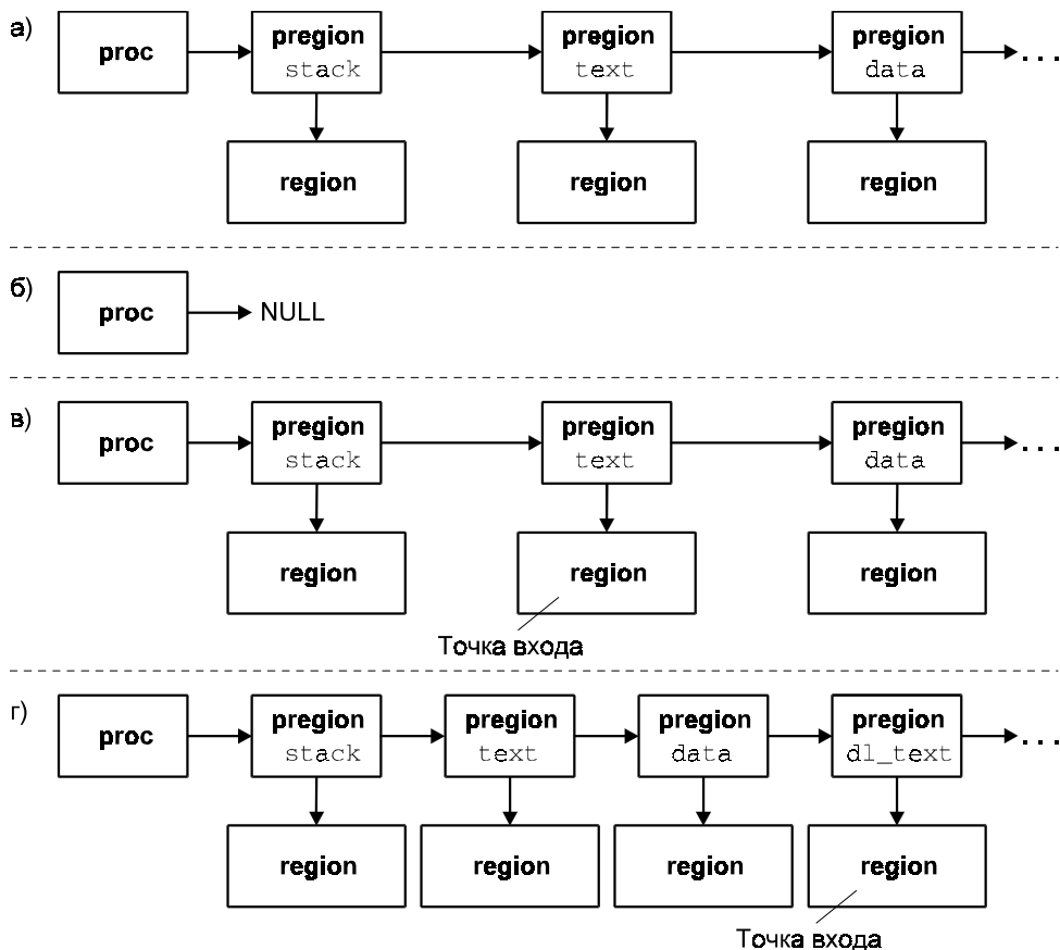
Рис. 3.16. Запуск новой программы: а) Адресное пространство процесса до вызова exec(2) ; б) Уничтожение старого адресного пространства; в) Новое адресное пространство процесса; г) Новое адресное пространство процесса при использовании динамических библиотек
