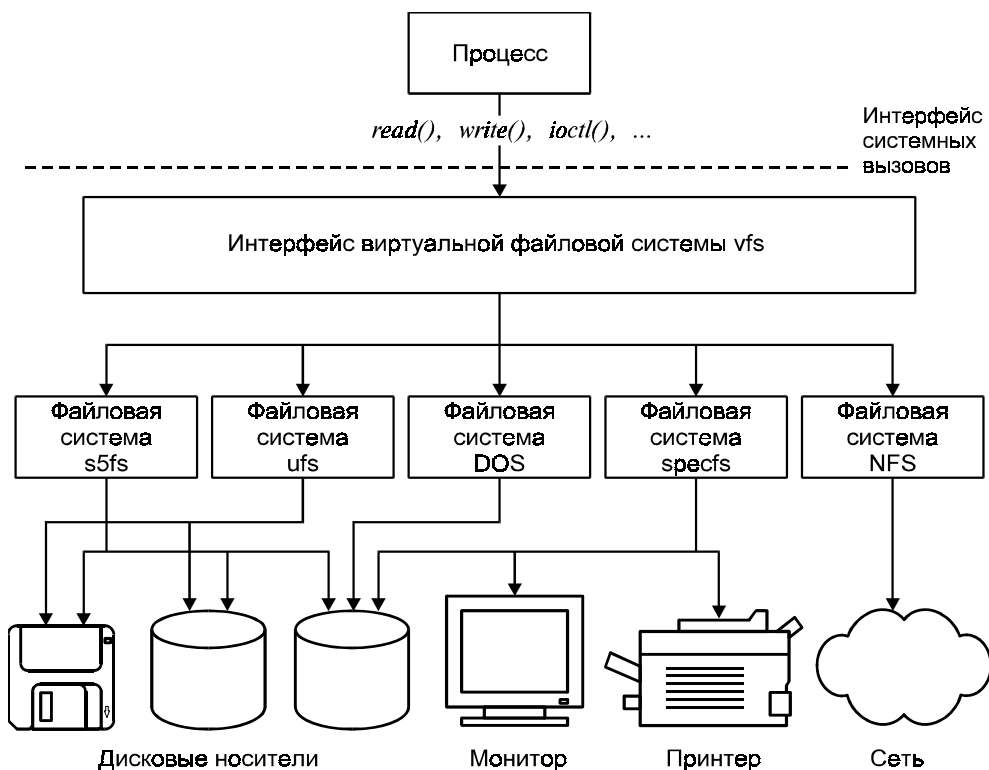
Рис. 4.7. Архитектура виртуальной файловой системы
