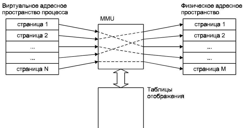
Рис. 3.4. Виртуальная и физическая память
