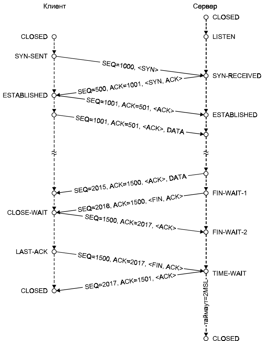
Рис. 6.20. Установление связи, передача данных и завершение TCP-сеанса
