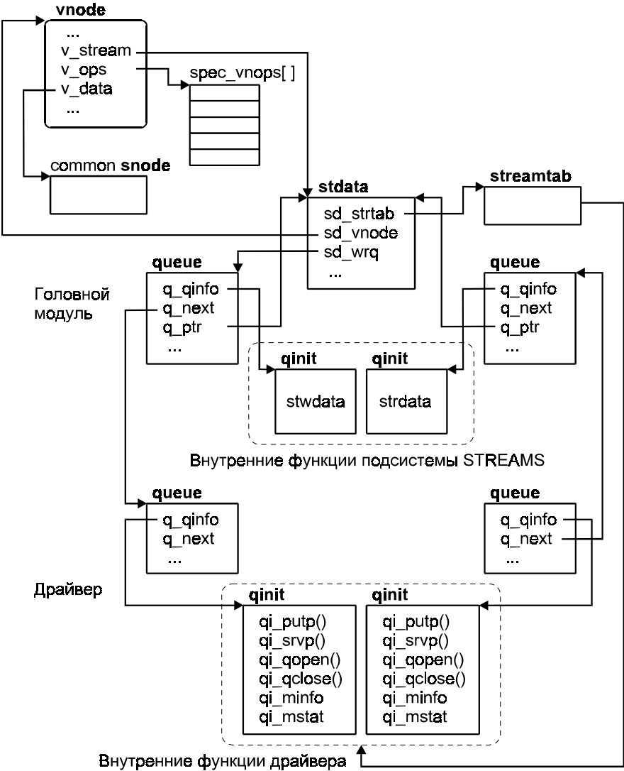
Рис. 5.22. Структура потока после открытия
