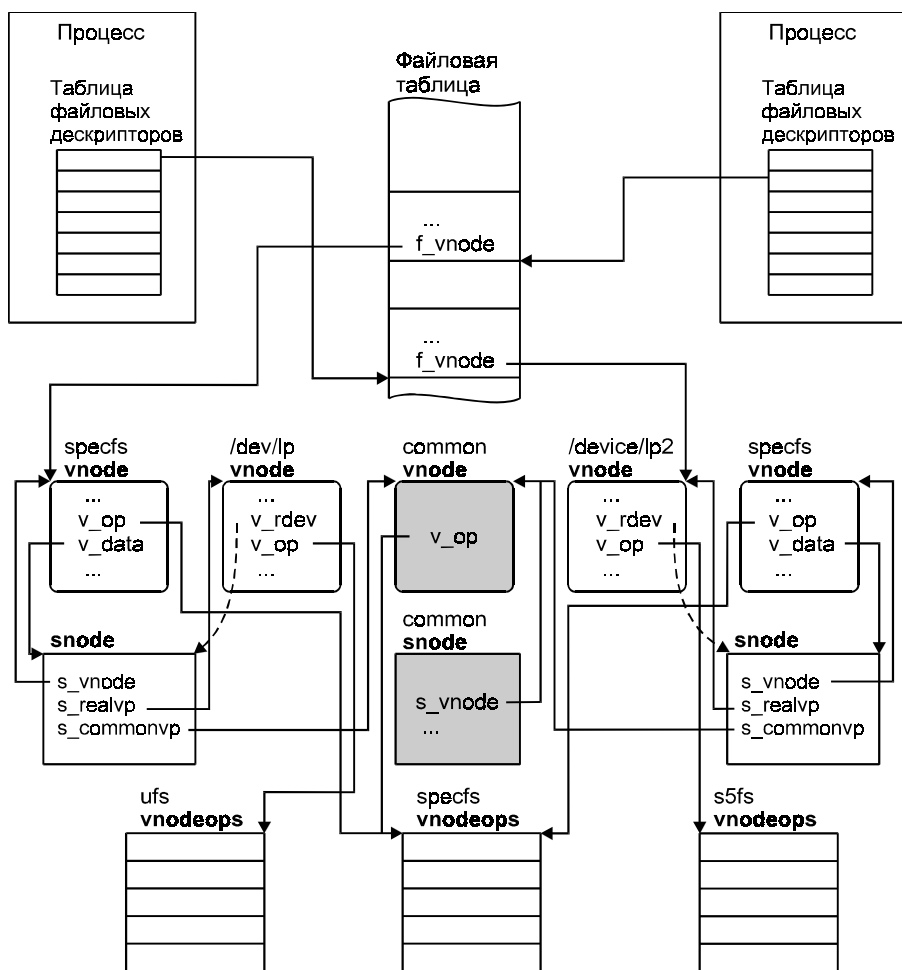
Рис. 5.5. Доступ к устройству через различные специальные файлы
