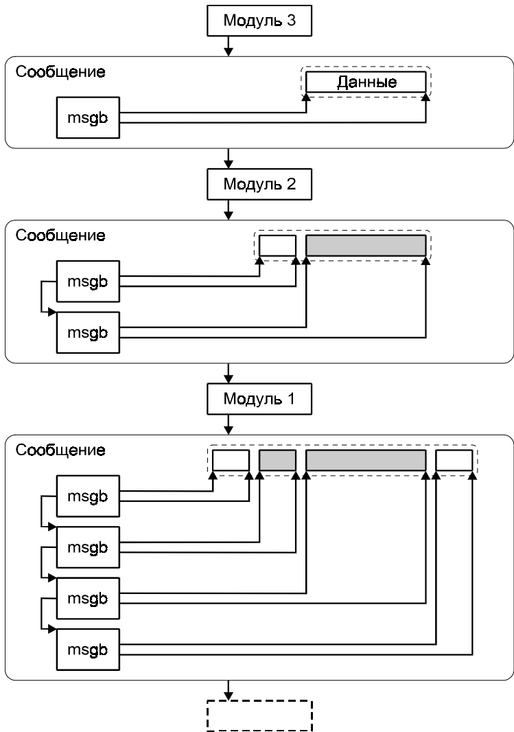
Рис. 5.18. Инкапсуляция данных с использованием составных сообщений
