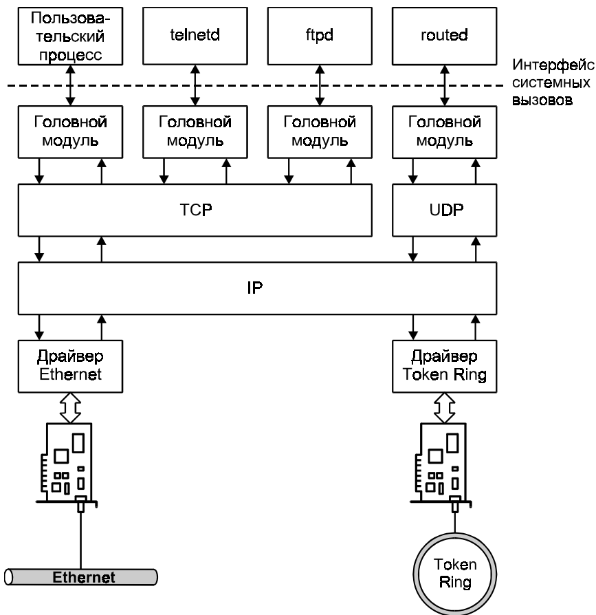
Рис. 5.15. Конфигурация сетевого доступа с использованием подсистемы STREAMS
