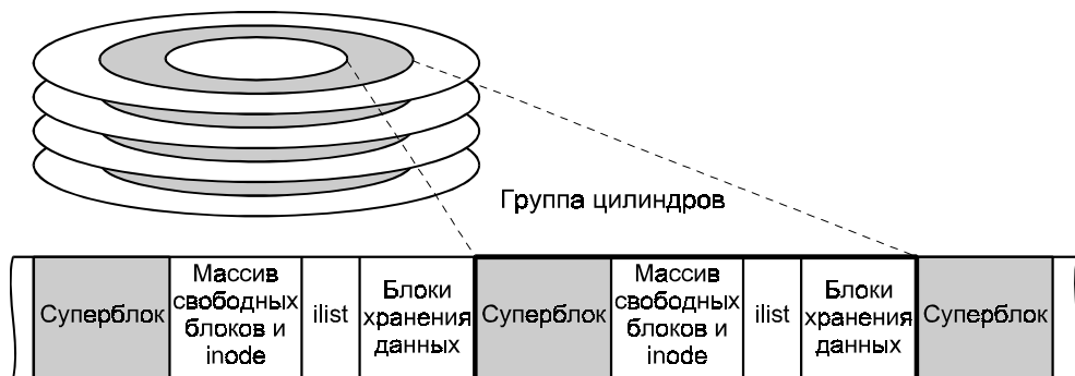
Рис. 4.4. Структура файловой системы FFS
