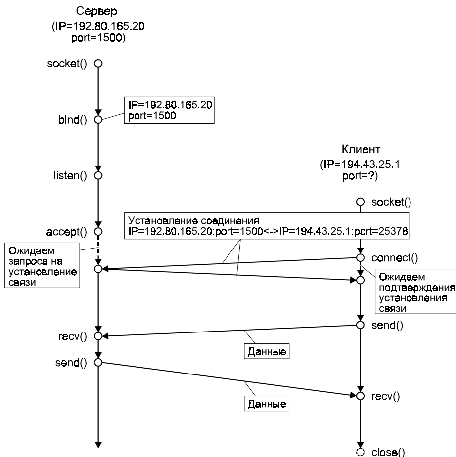
Рис. 6.25. Схема установления связи и передачи данных между клиентом и сервером
