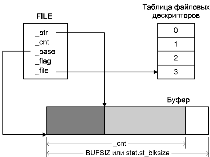
Рис. 2.9. Структуры данных потока
