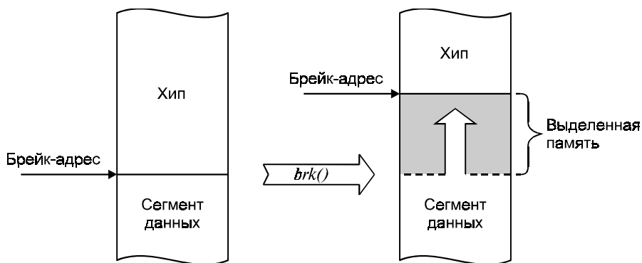
Рис. 2.11. Динамическое выделение памяти с помощью brk(2)
