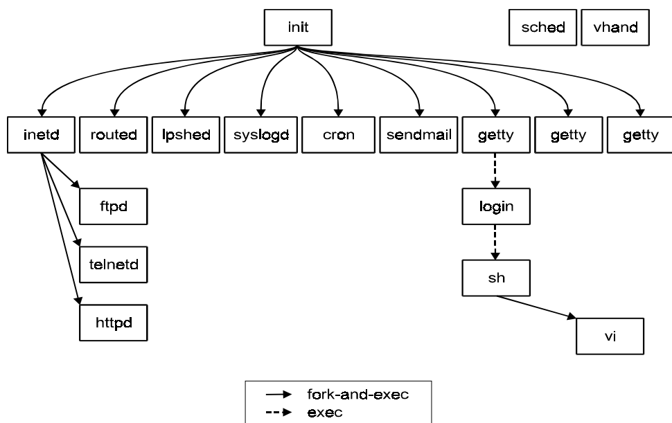
Рис. 1.6. Типичное "дерево" процессов в UNIX
