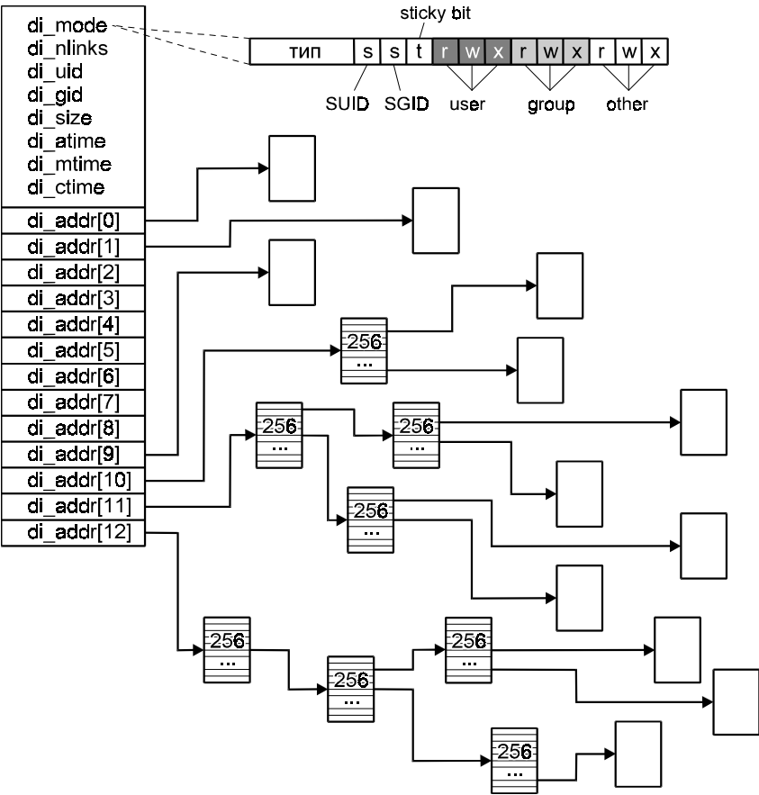
Рис. 4.2. Структура индексного дескриптора на диске
