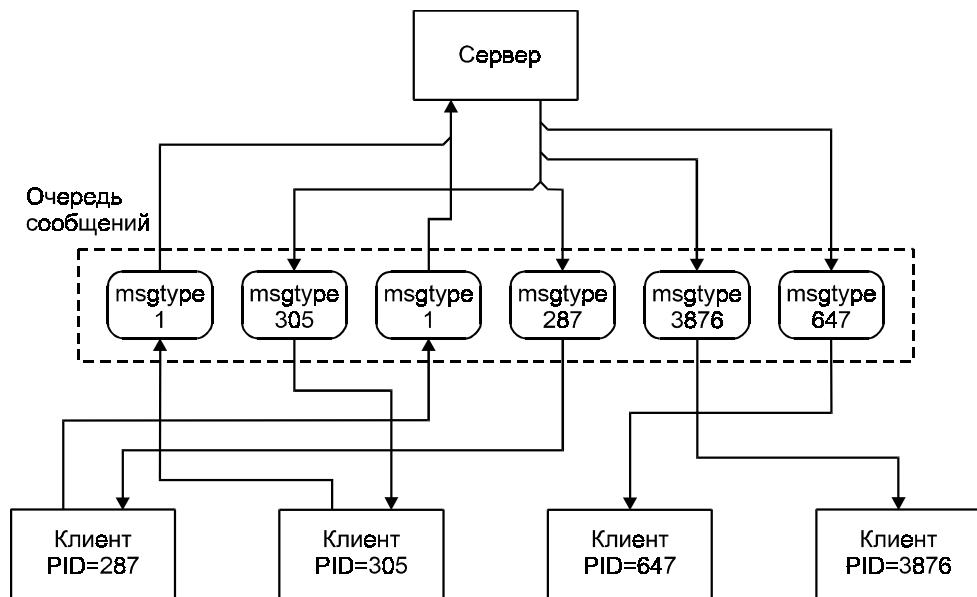
Рис. 3.19. Мультиплексирование сообщений в одной очереди
