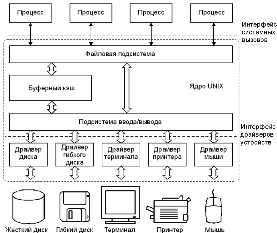
Рис. 5.1. Драйверы устройств UNIX
