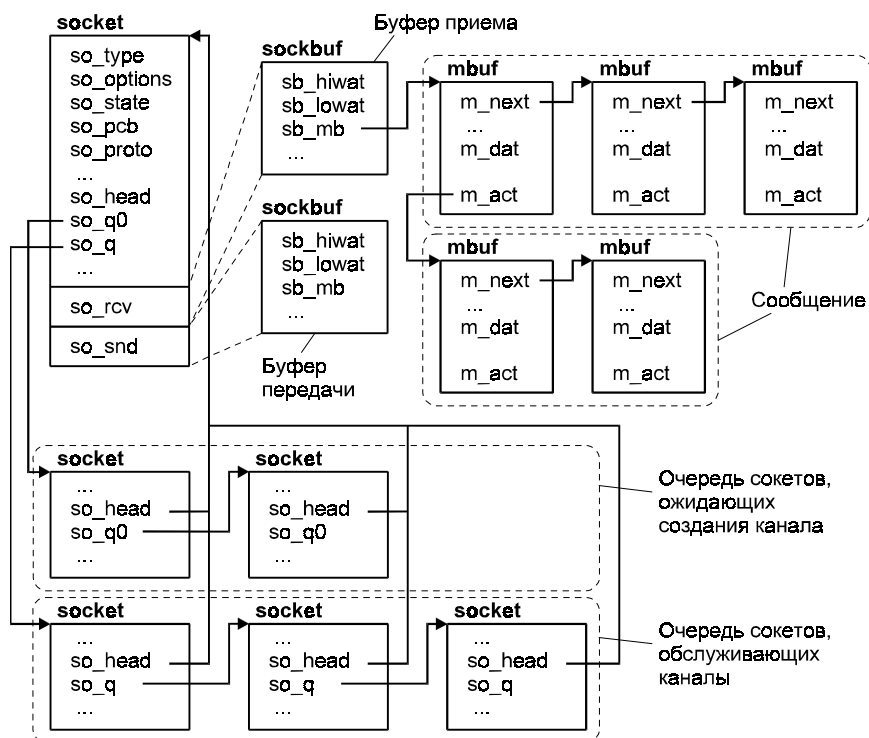
Рис. 6.29. Структуры данных сокета
