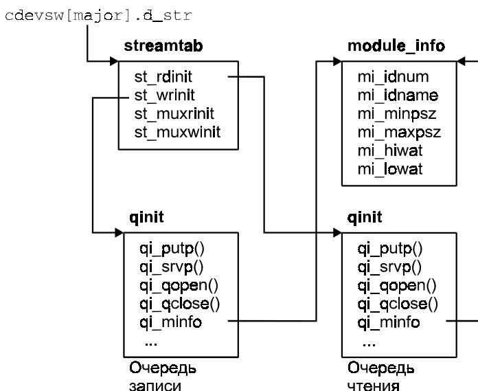
Рис. 5.21. Конфигурационные данные драйвера (модуля) STREAMS
