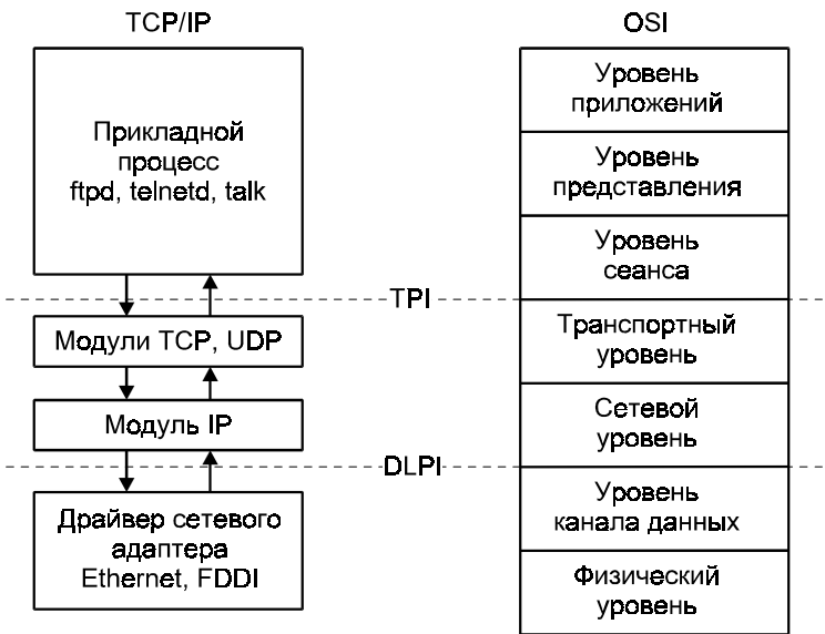
Рис. 6.39. Интерфейсы взаимодействия модулей протоколов
