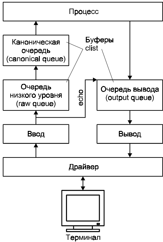
Рис. 5.10. Пример использования буферов структуры clist в драйвере терминала
