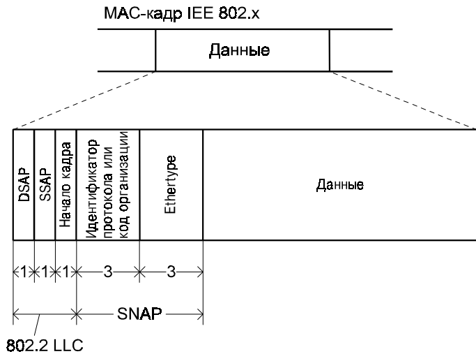
Рис. 6.47. Формат кадра LLC
