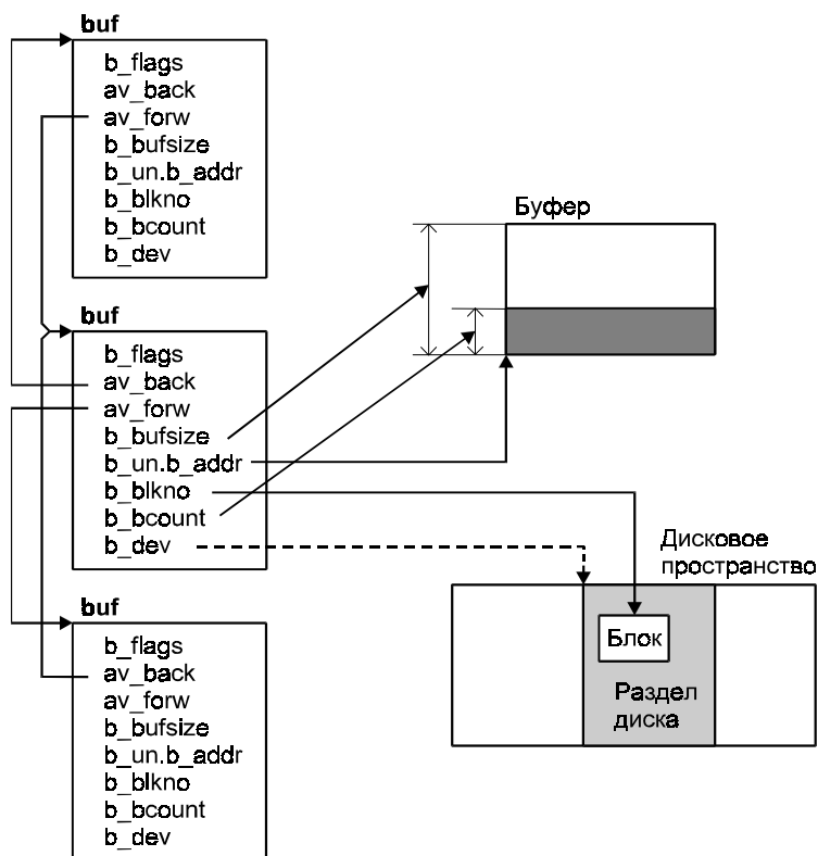
Рис. 5.7. Обмен данными с блочным устройством (диском)
