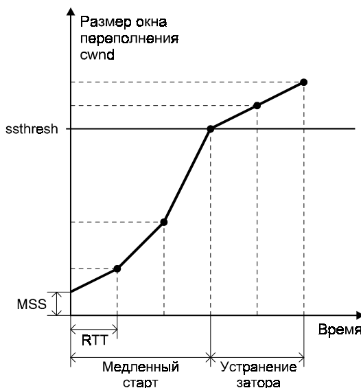
Рис. 6.24. Рост окна переполнения при медленном старте и устранении затора
