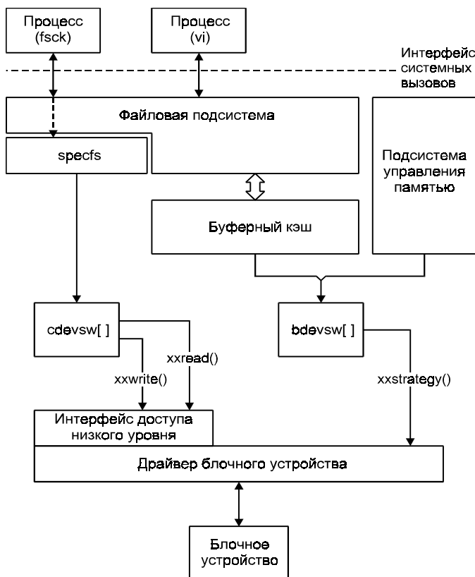
Рис. 5.8. Различные типы доступа к блочным устройствам
