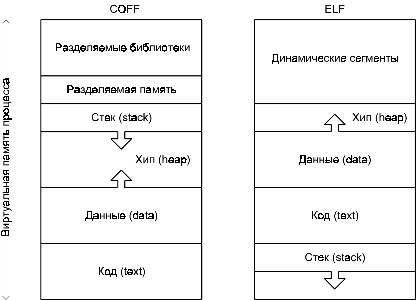
Рис. 2.3. Исполняемые образы программ форматов COFF и ELF
