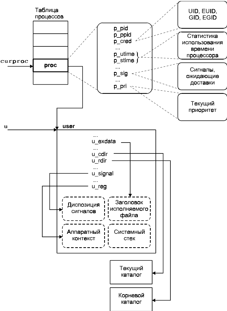
Рис. 3.2. Основные структуры данных процесса
