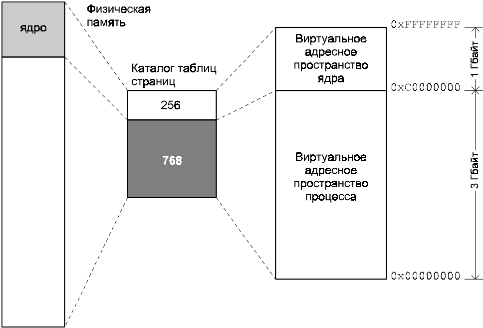
Рис. 3.8. Адресное пространство в режимах ядра и задачи
