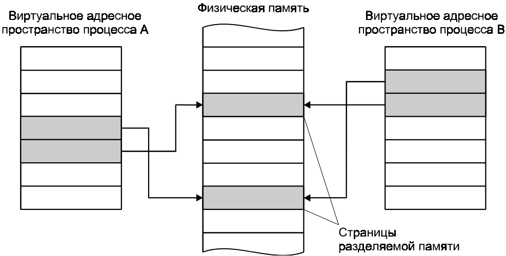
Рис. 3.20. Совместное использование разделяемой памяти
