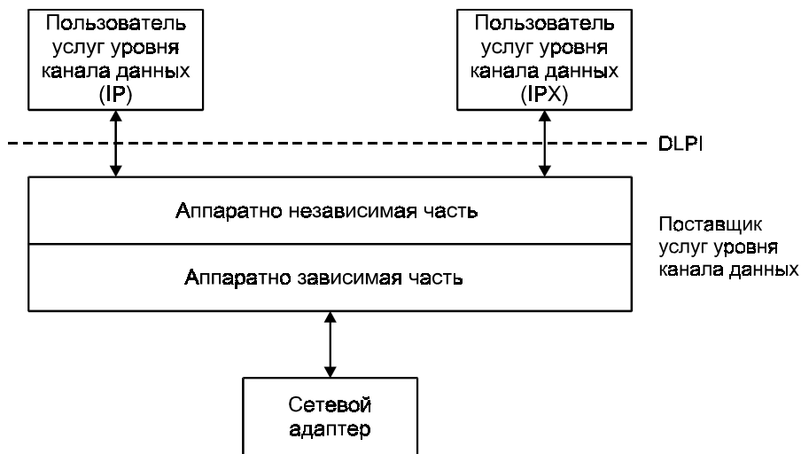
Рис. 6.42. Структура драйвера уровня канала данных
