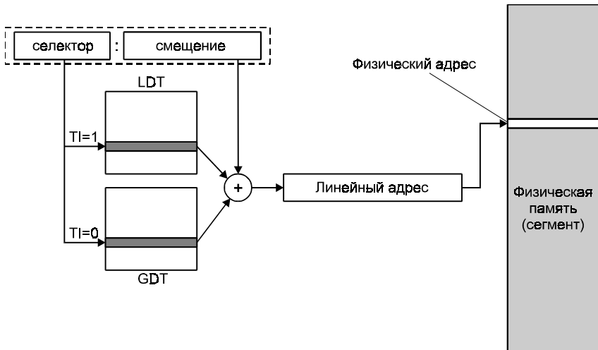
Рис. 3.6. Трансляция адреса с использованием механизма сегментации
