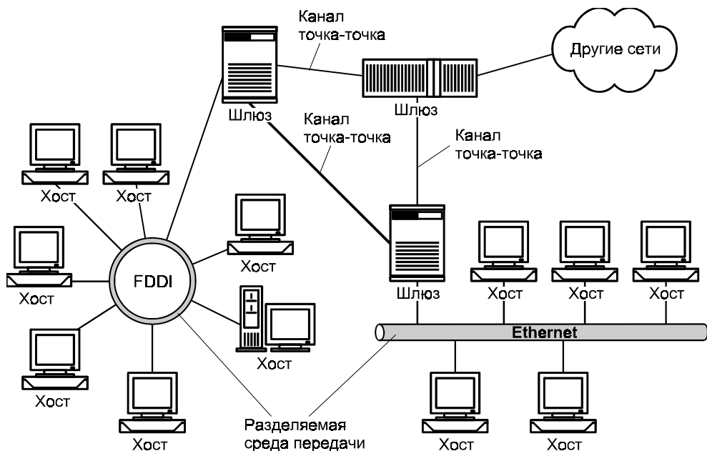
Рис. 6.32. Коммуникационная среда UNIX (internetwork)
