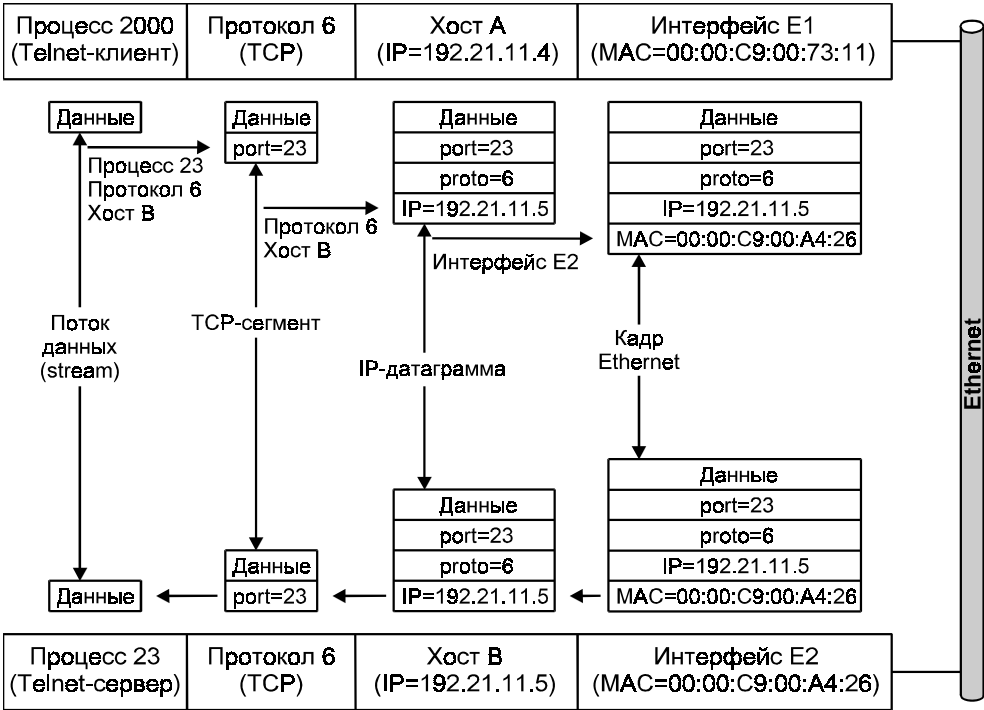
Рис. 6.3. Обработка данных в соответствии с протоколами TCP/IP
