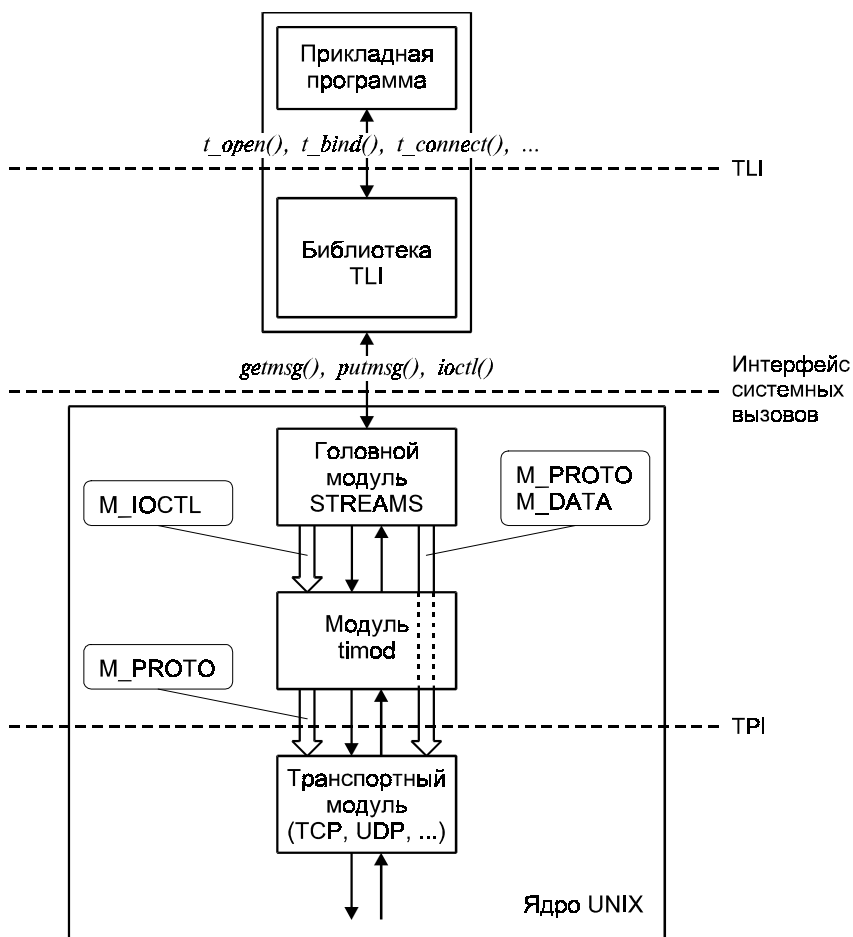
Рис. 6.41. Архитектура доступа к транспортным услугам
