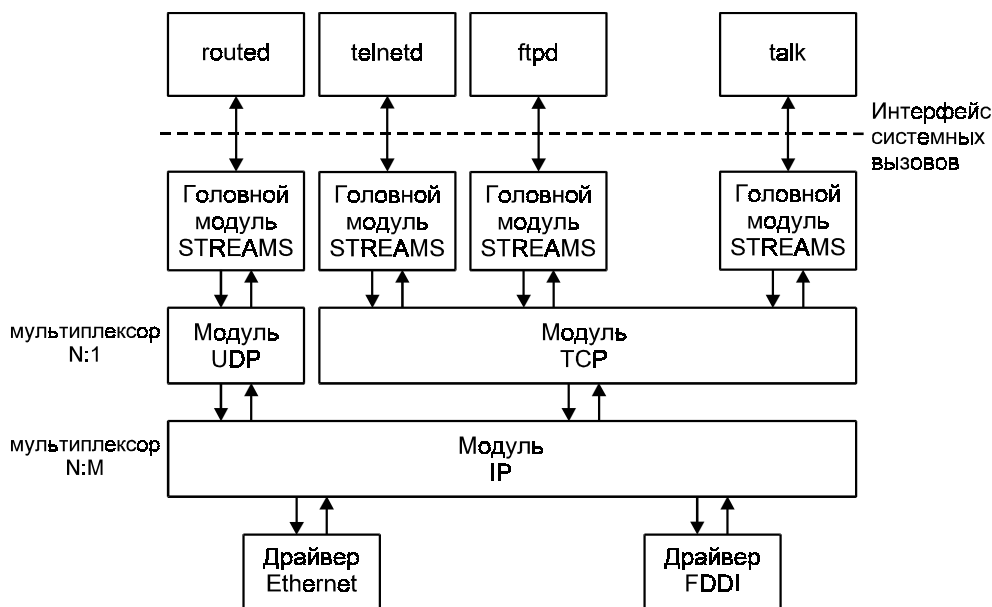
Рис. 6.38. Реализация протоколов TCP/IP на основе архитектуры STREAMS
