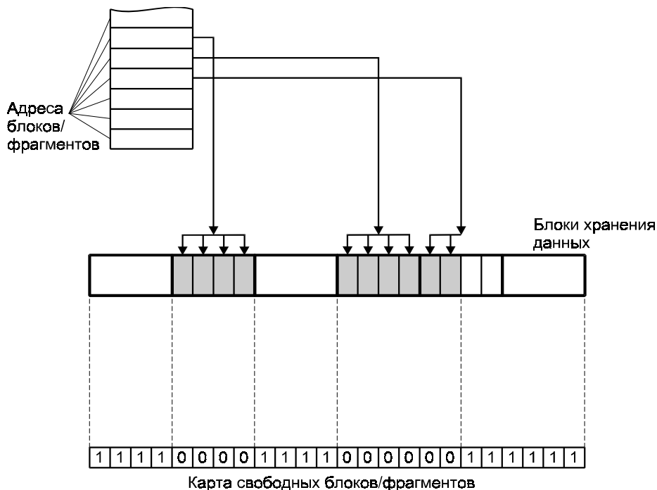
Рис. 4.5. Карта свободных блоков
