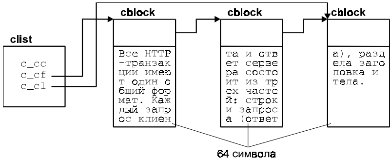
Рис. 5.9. Буферизация данных с помощью структуры clist
