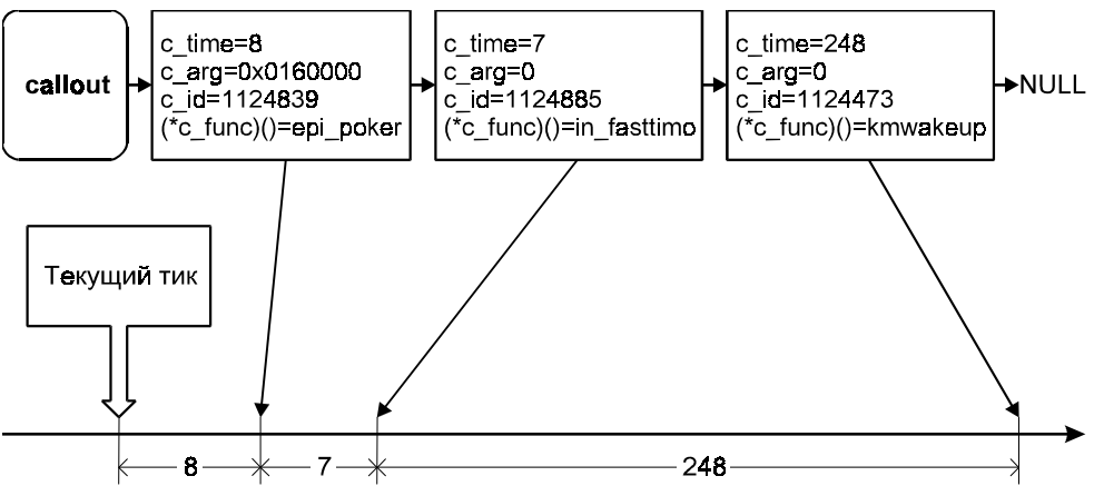
Рис. 3.14. Организация таблицы отложенных вызовов
