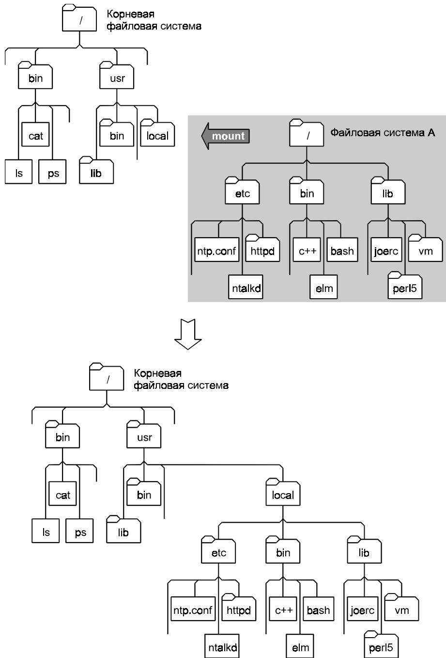
Рис. 4.10. Монтирование файловой системы А к корневой файловой системе
