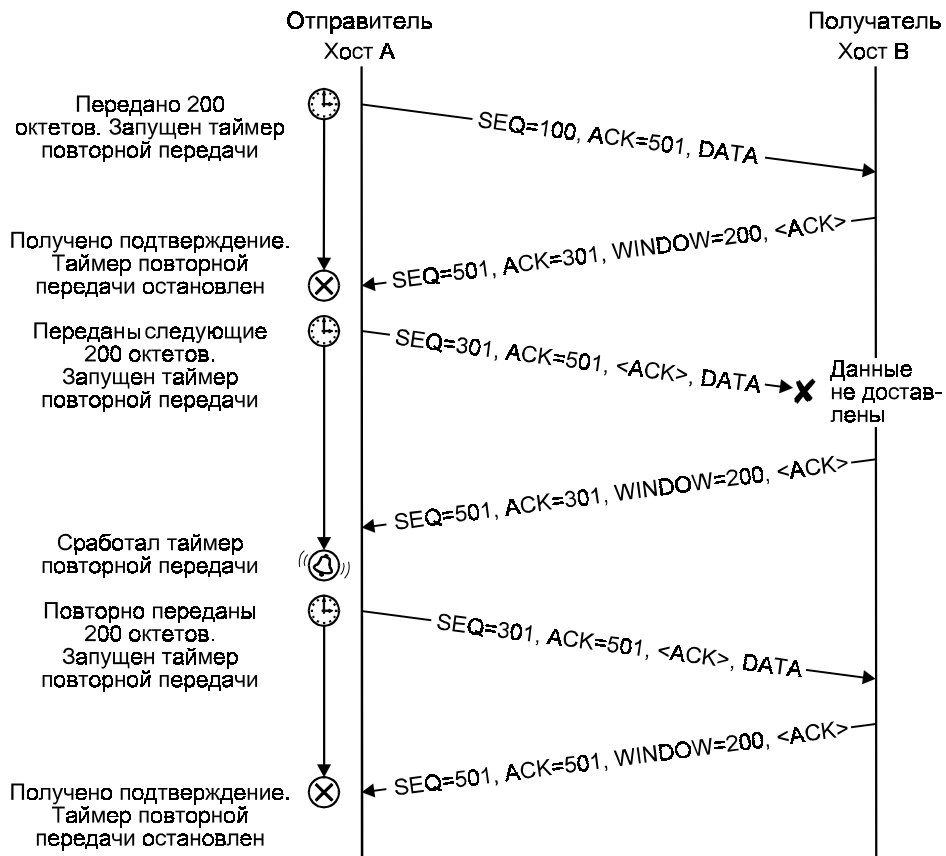
Рис. 6.21. Повторная передача
