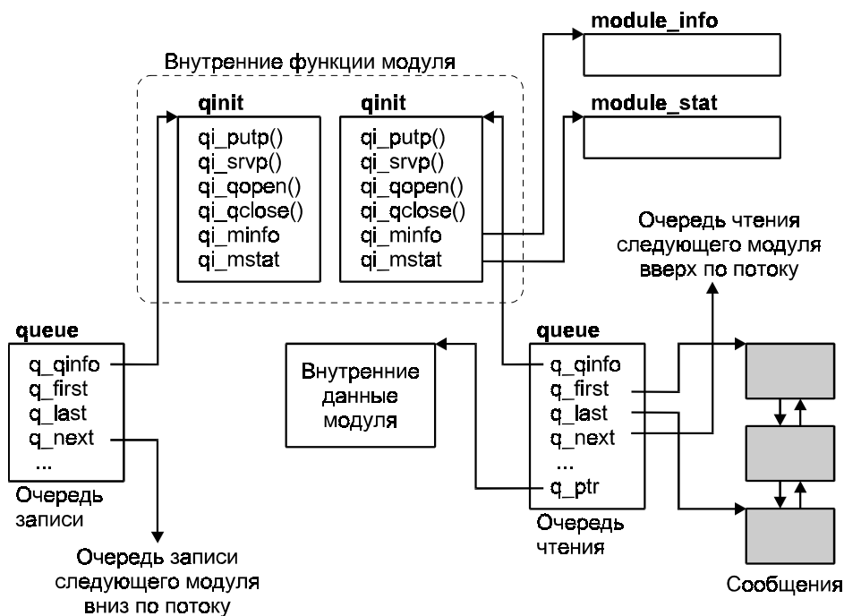
Рис. 5.16. Модуль STREAMS
