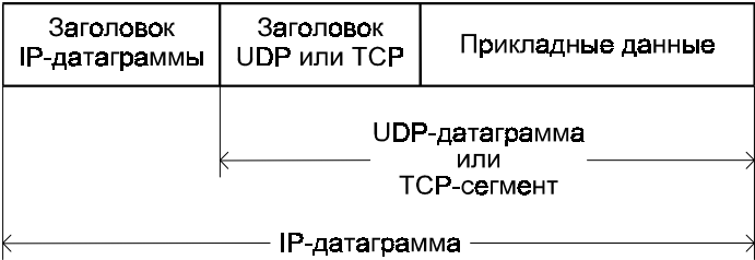
Рис. 6.5. IP-датаграмма
