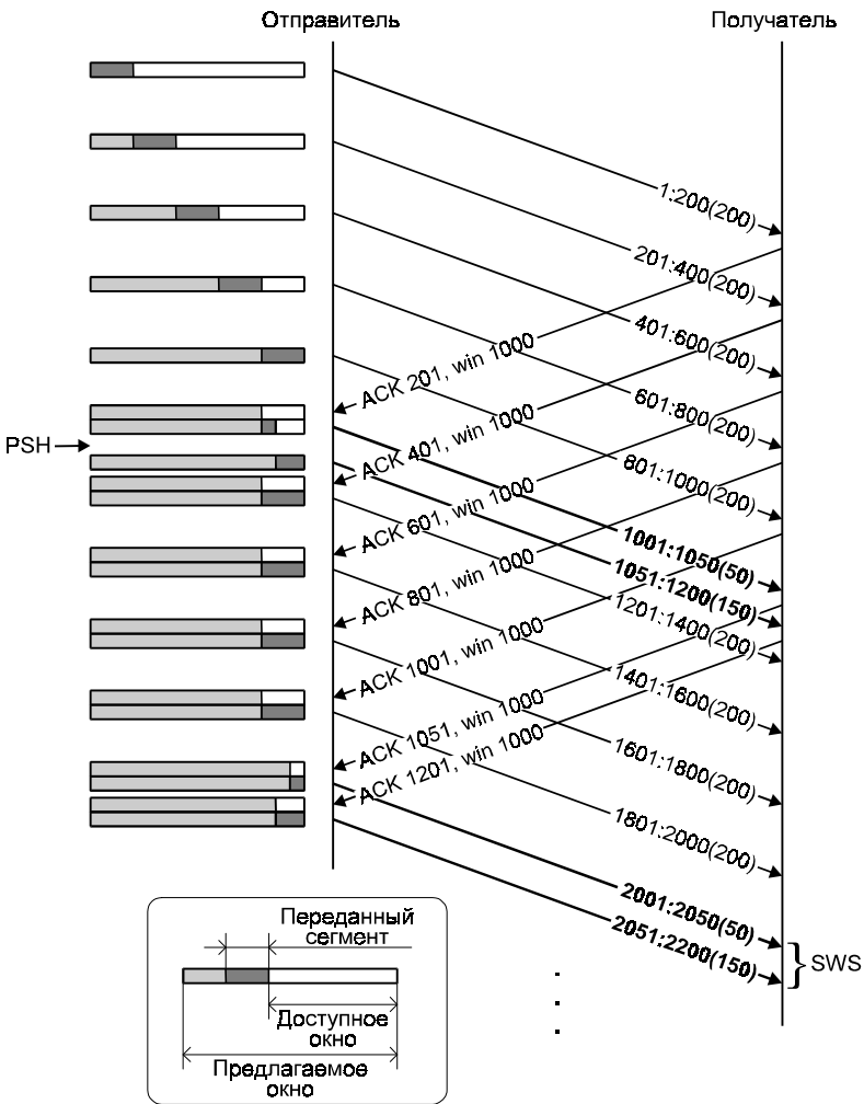
Рис. 6.23. Возникновение SWS
