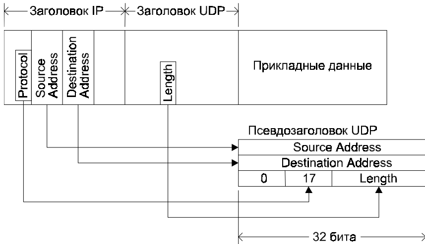
Рис. 6.18. Псевдозаголовок UDP
