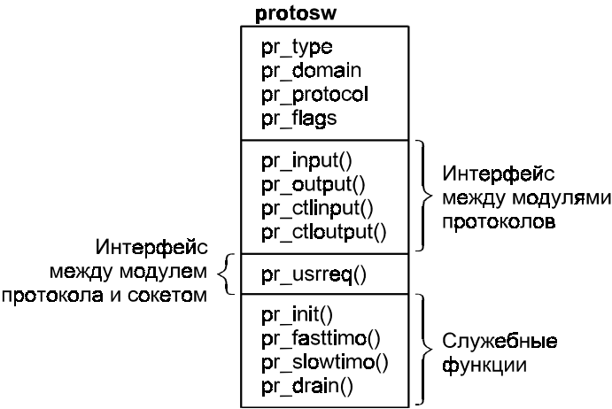
Рис. 6.30. Коммутатор протокола
