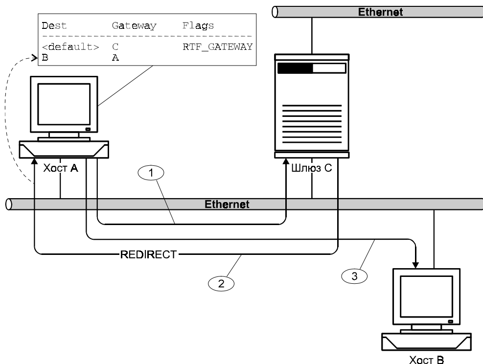
Рис. 6.35. Перенаправление маршрутов
