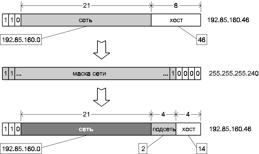
Рис. 6.8. Подсети
