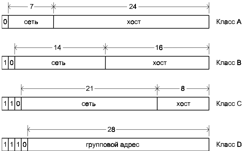
Рис. 6.7. Форматы IP-адресов
