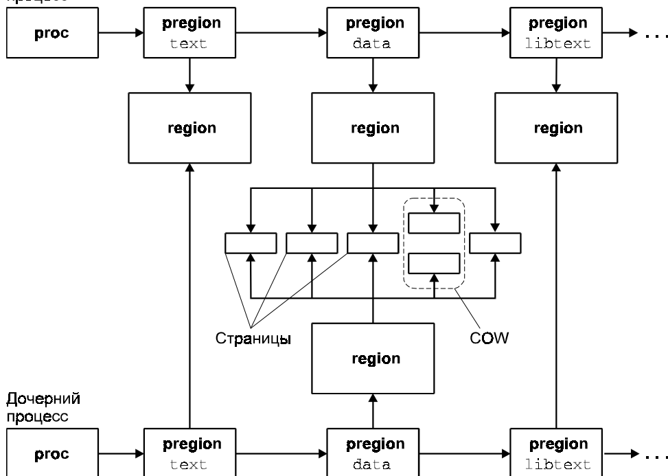
Рис. 3.15. Создание областей нового процесса
