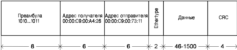
Рис. 6.44. Формат кадра Ethernet
