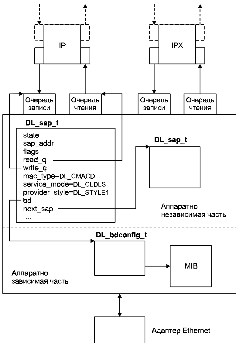
Рис. 6.48. Архитектура драйвера DLPI
