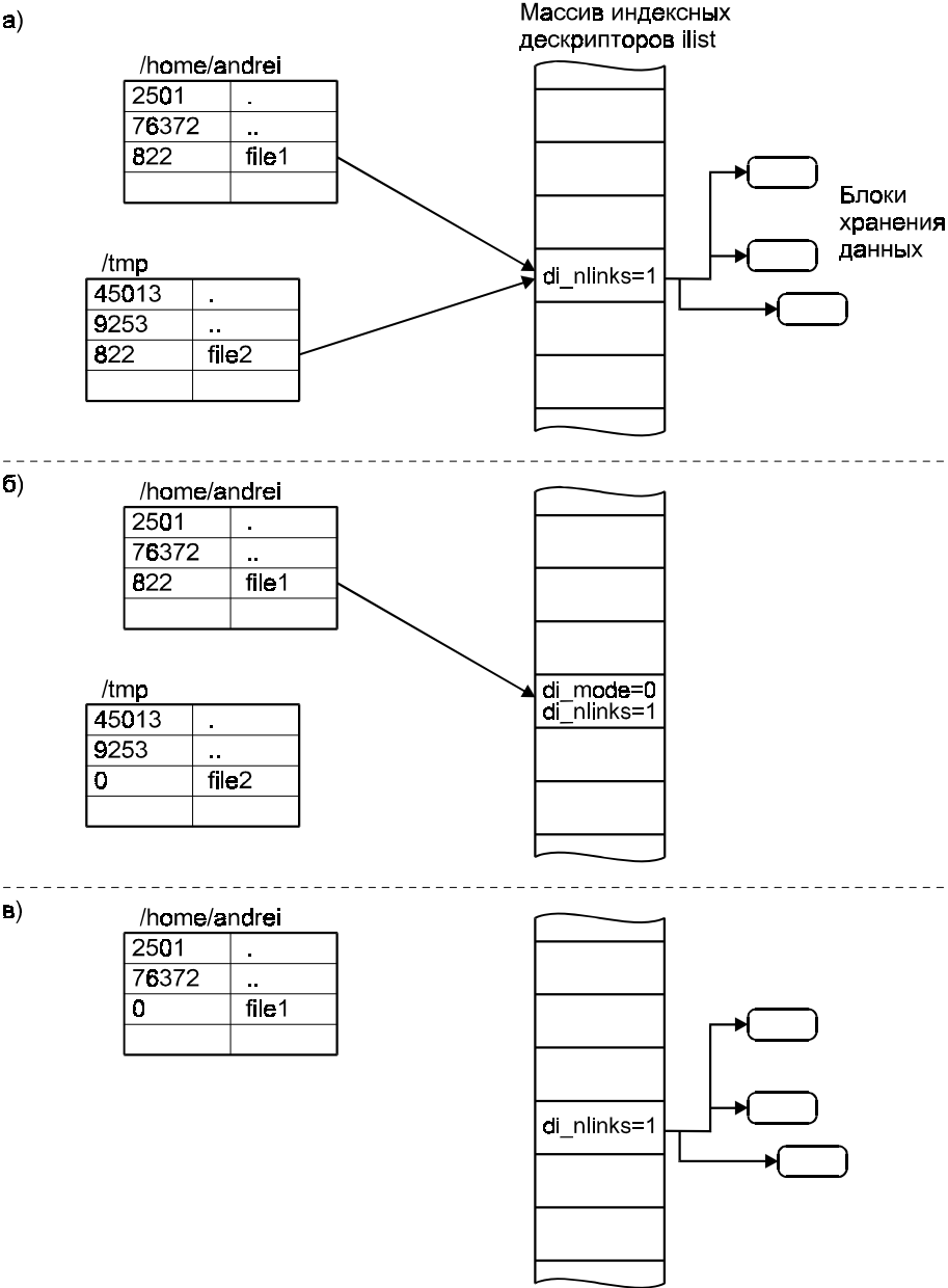
Рис. 4.15. Нарушение целостности файловой системы
