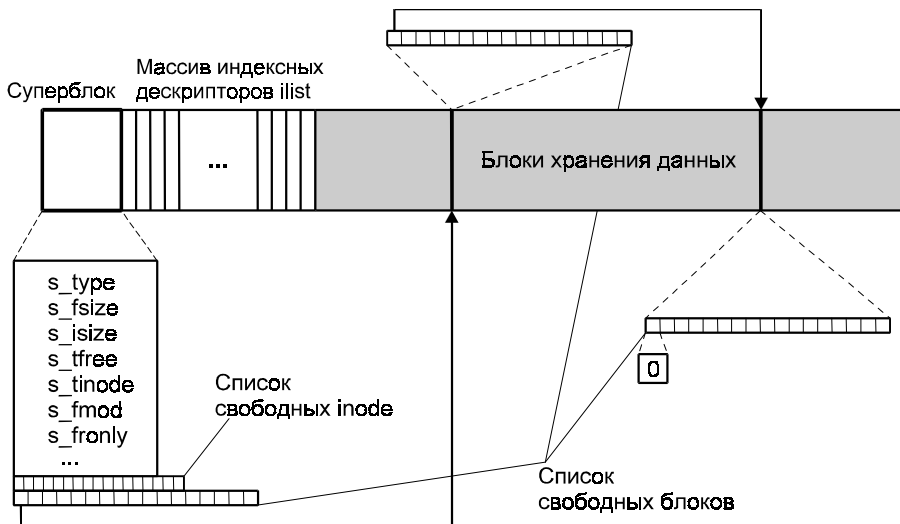
Рис. 4.1. Структура файловой системы s5fs
