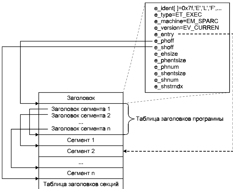
Рис. 2.4. Структура исполняемого файла в формате ELF
