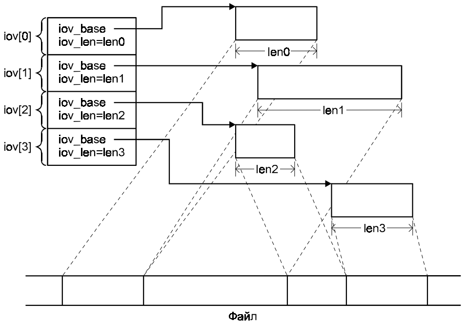
Рис. 2.8. Чтение файла с использованием нескольких буферов
