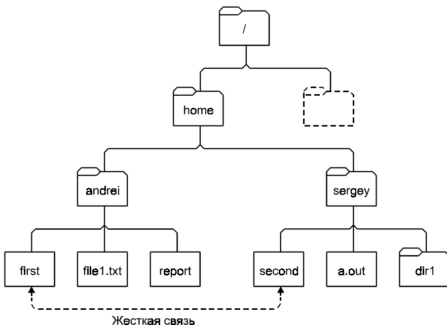
Рис. 1.2. Структура файловой системы после выполнения команды ln (1) . Жесткая связь имен с данными файла
