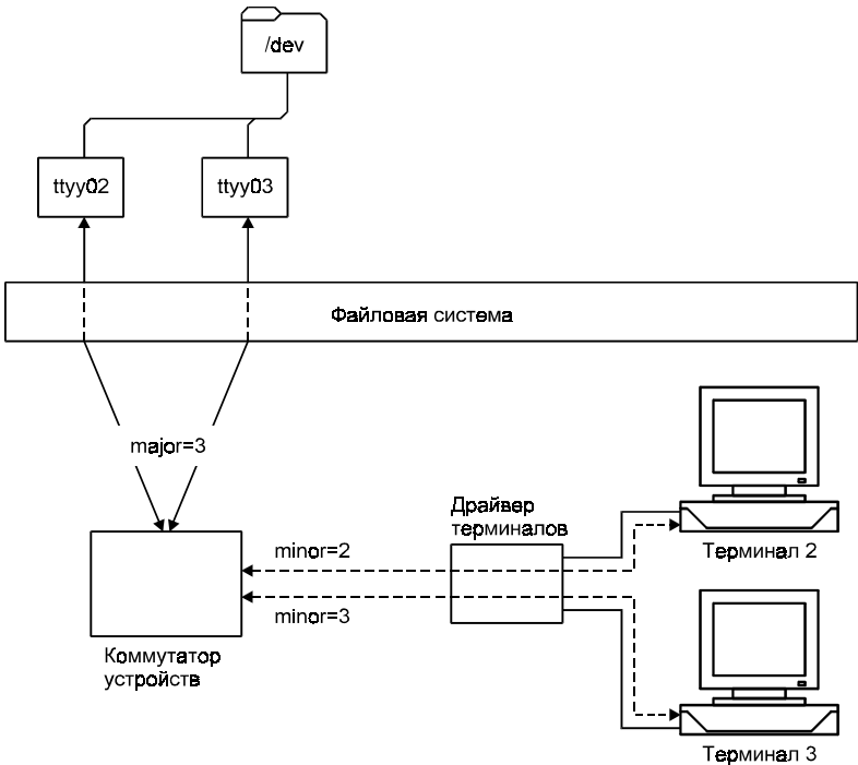
Рис. 1.7. Взаимодействие файловой системы с устройством
