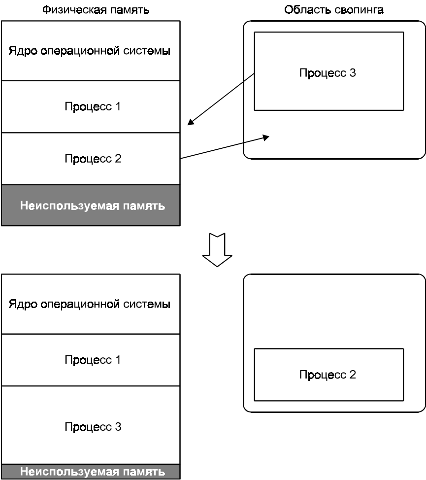
Рис. 3.11. Управление памятью, основанное на свопинге
