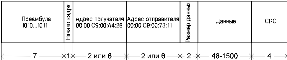
Рис. 6.45. Формат кадра IEEE 802.3
