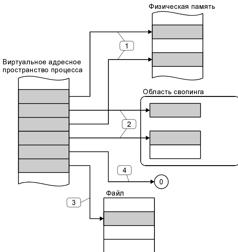
Рис. 3.13. Возможное местонахождение физических страниц процесса
