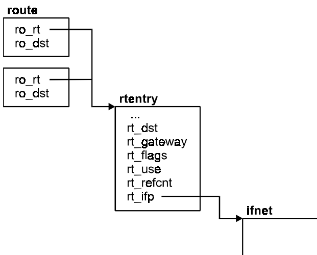
Рис. 6.33. Элемент таблицы маршрутизации
