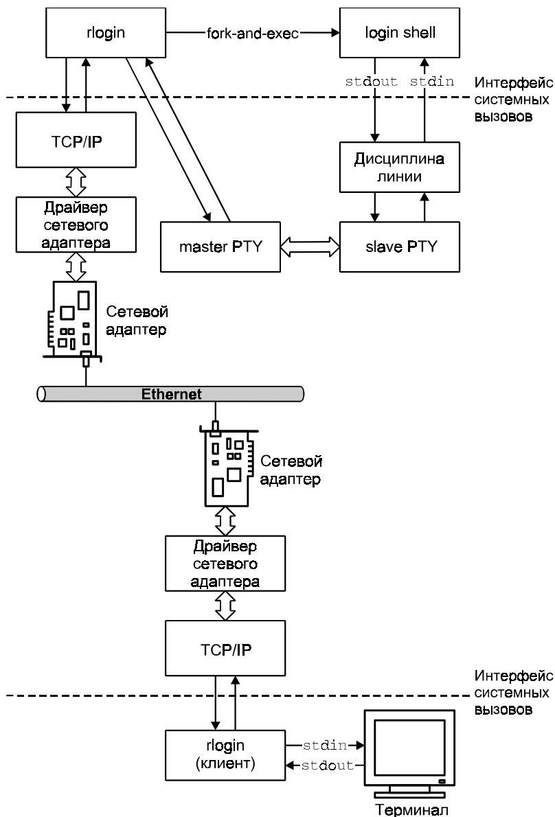
Рис. 5.12. Архитектура удаленного доступа с использованием псевдотерминала
