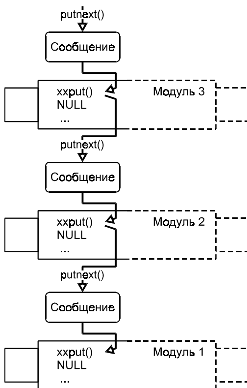
Рис. 5.19. Передача данных без управления потоком
