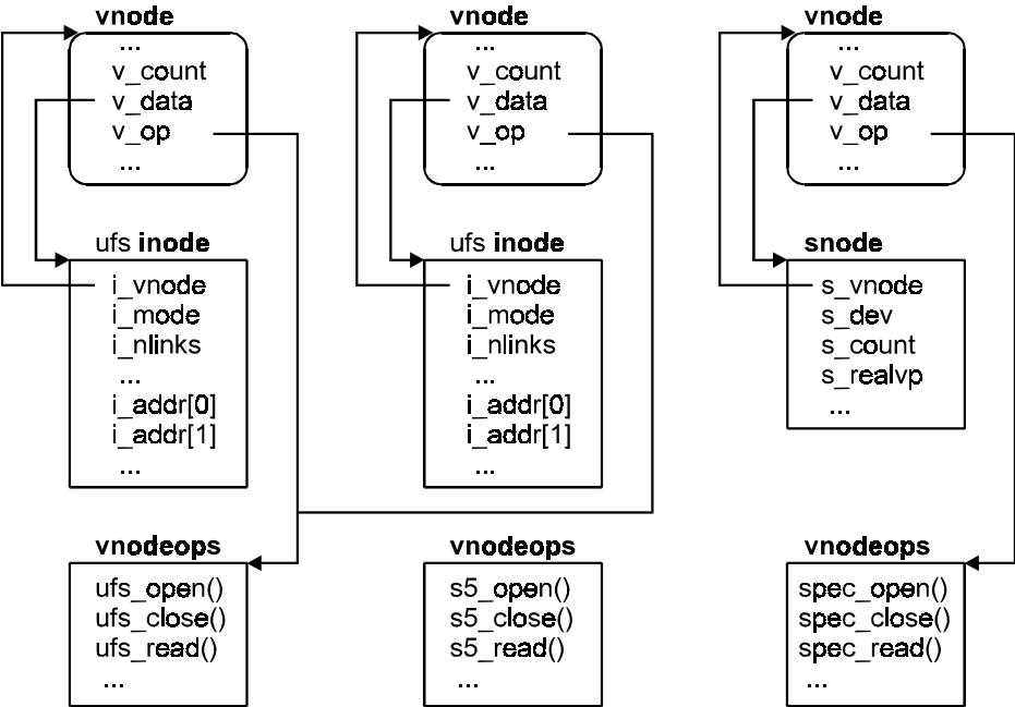
Рис. 4.8. Метаданные файла виртуальной файловой системы
