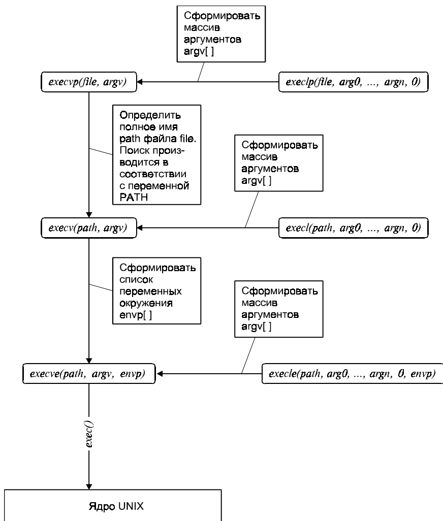
Рис. 2.12. Семейство функций \text{exes}(2)
