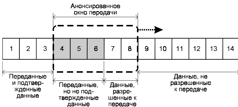
Рис. 6.22. Окно передачи TCP
