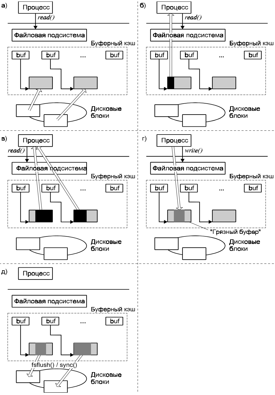
Рис. 4.14. Схема работы буферного кэша
