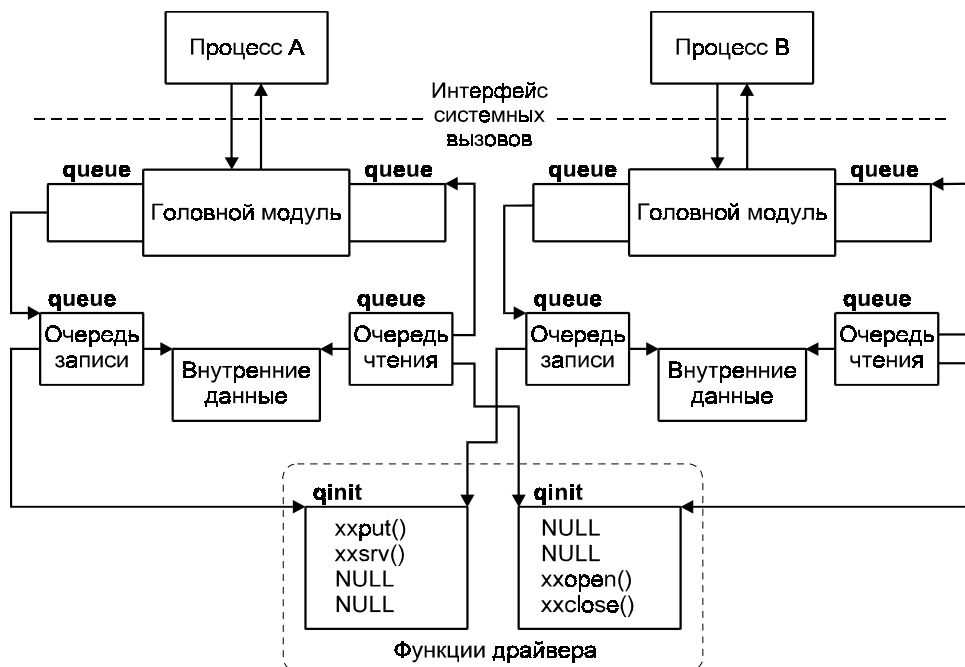
Рис. 5.23. Верхний мультиплексор
