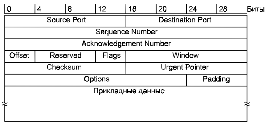
Рис. 6.19. Формат TCP-сегмента
