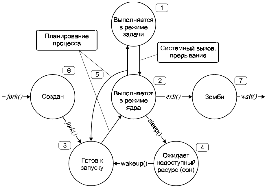
Рис. 3.3. Состояния процесса
