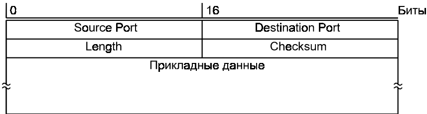
Рис. 6.17. Заголовок UDP
