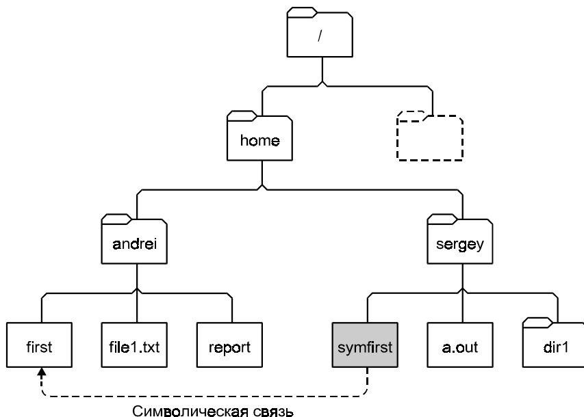
Рис. 1.3. Символическая связь
