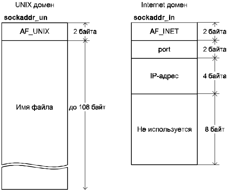
Рис. 3.23. Адреса сокетов
