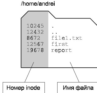
Рис. 1.1. Структура каталога
