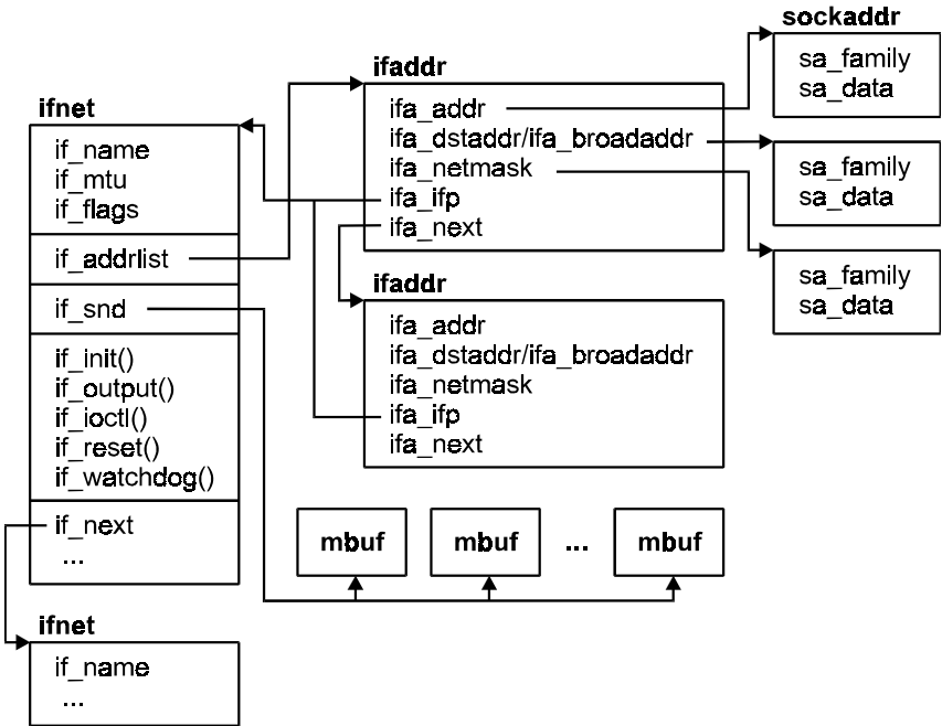
Рис. 6.31. Сетевой интерфейс
