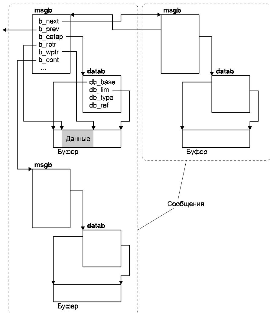
Рис. 5.17. Сообщения STREAMS
