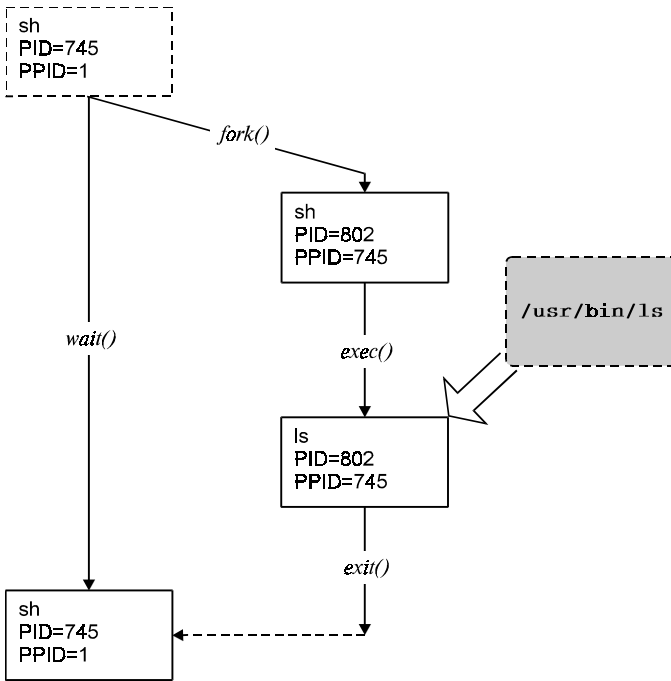
Рис. 1.5. Создание процесса и запуск программы
