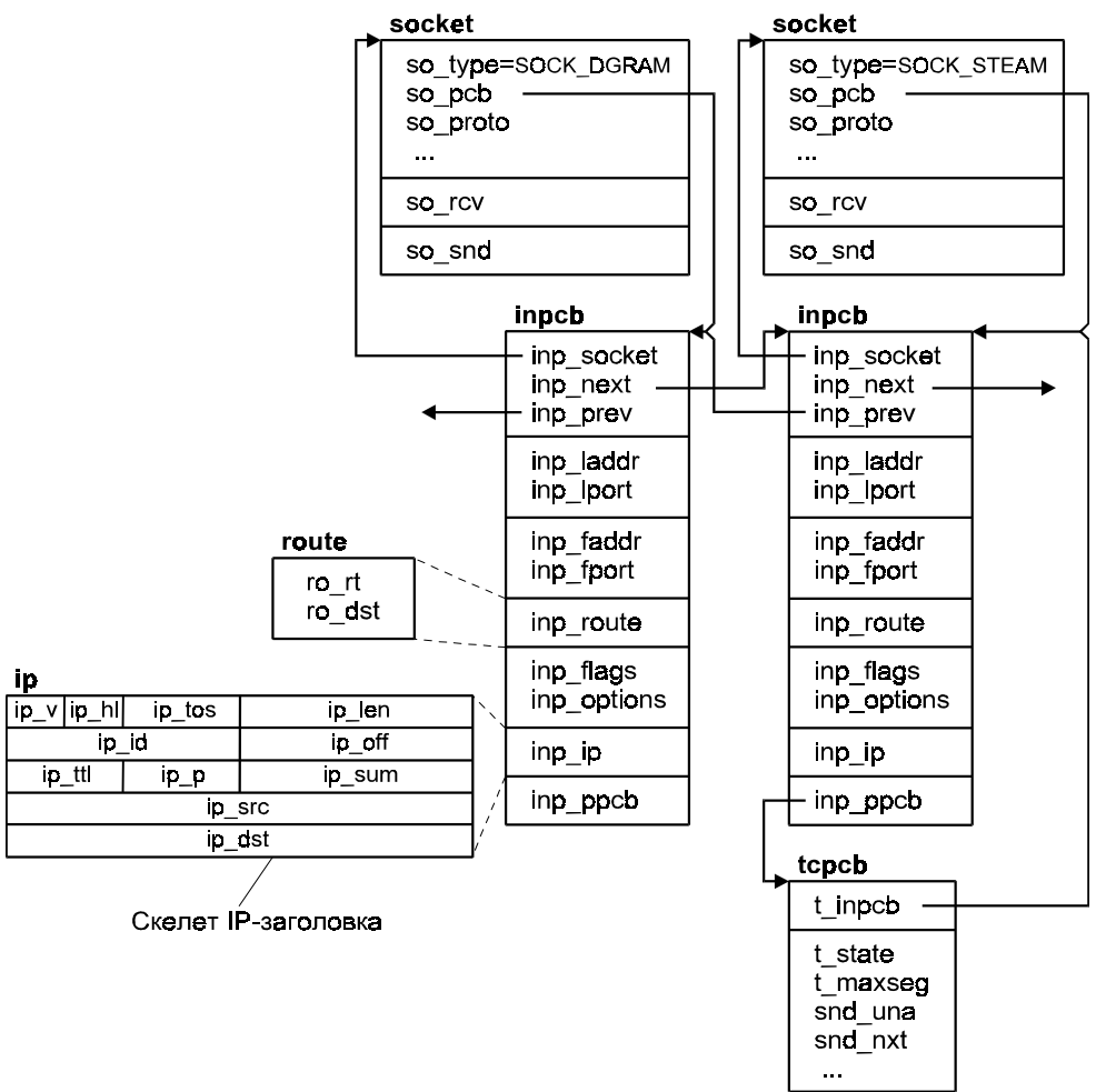
Рис. 6.36. Структуры данных протоколов TCP/IP
