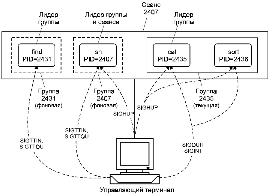
Рис. 2.13. Связь между управляющим терминалом, сеансом и группами
